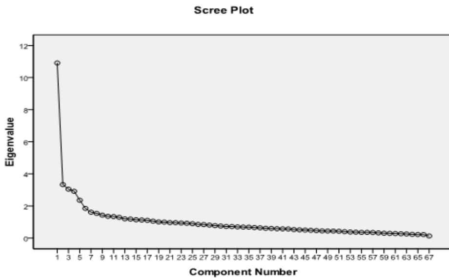
Şekil 6 Scree Plot
