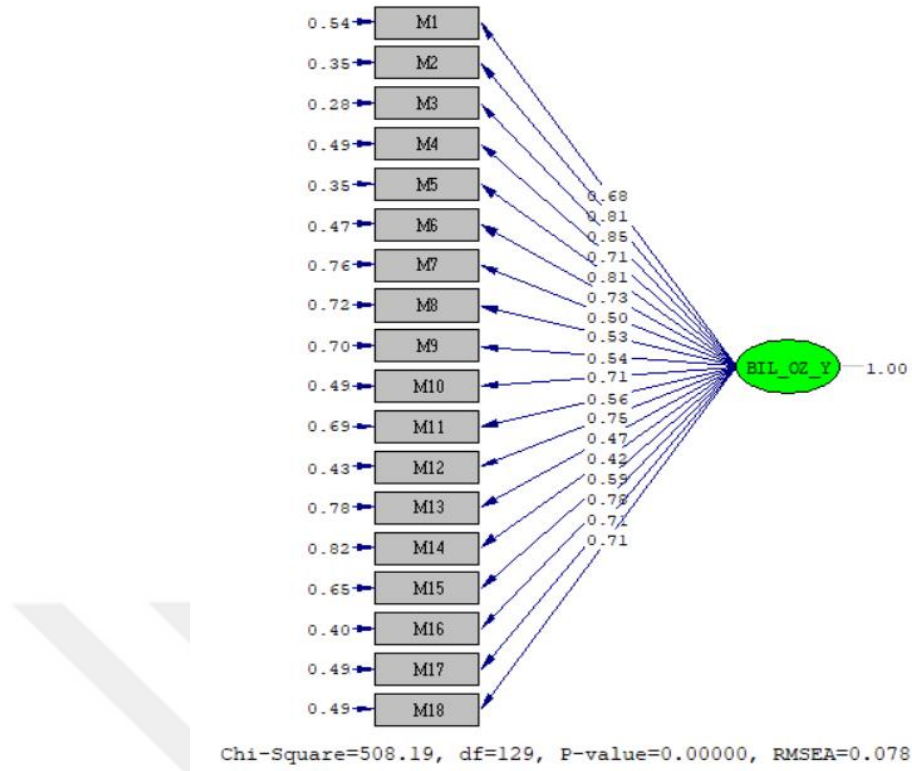
Şekil 1. Bilgisayara İlişkin Öz Yeterlilik Algısı Ölçeğine Ait DFA Path Diagramı
