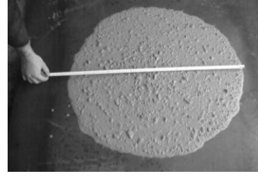
Şekil 1. Kendiliğinden yerleşen beton için çökme-yayılma ve T_{50} testleri
