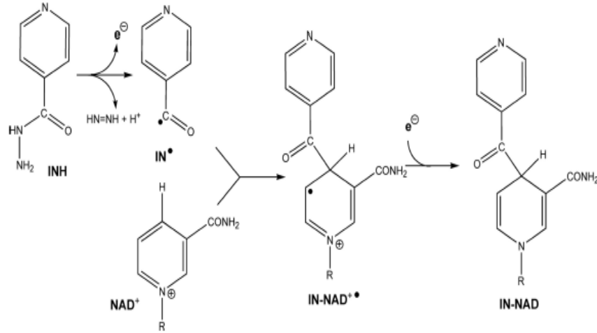
Şekil 2.7. İzoniyazidin aktivasyonu (48)
