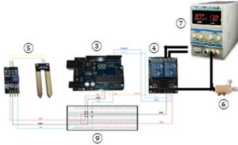
Şekil 9. Toprak Nem Ölçme Sensörlü Otomatik Çiçek Sulama Şeması Genel Görünümü
