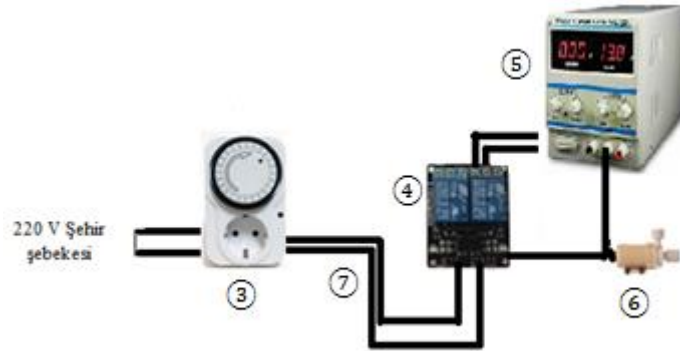
Şekil 11. Mekanik Zaman Ayarlı Otomatik Çiçek Sulama Sistemi Şeması Genel Görünümü
