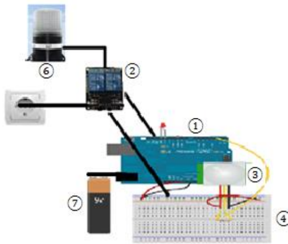
Şekil 18. Arduino Pır Hareket Sensörlü Hırsız Alarm Devresi Genel Görünümü
