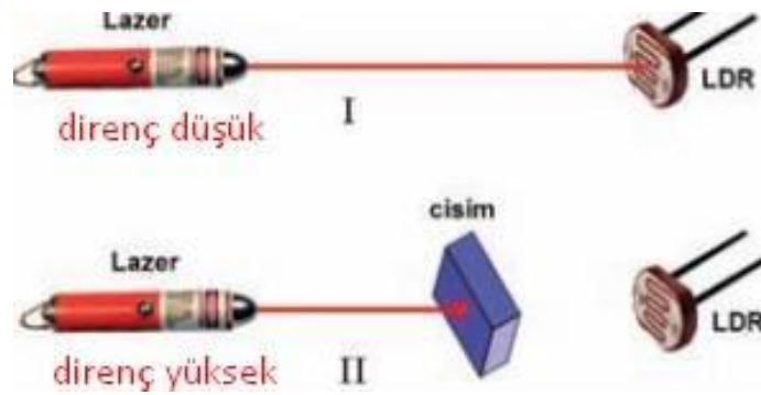
Şekil 20. Elektronik Işık Sensörlü Hırsız Alarm Şeması Genel Görünümü
