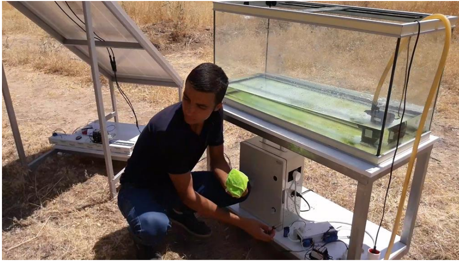
Şekil 4. Güneş Enerjili, Toprak Nem Ölçme Sensörlü Otomatik Kayısı Sulama Sistemi Uygulaması
