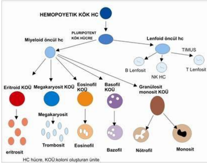
Şekil 1.Hematopoez
