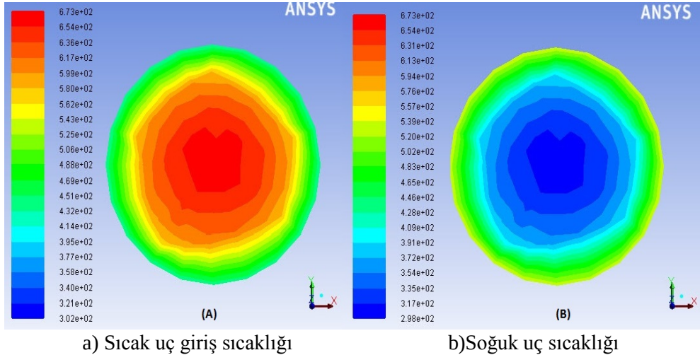
Şekil 4.13. 673^{\circ}\text{K} Demir'den imal displacer borusunun sıcak uç giriş ve soğuk uç sıcaklıkları
