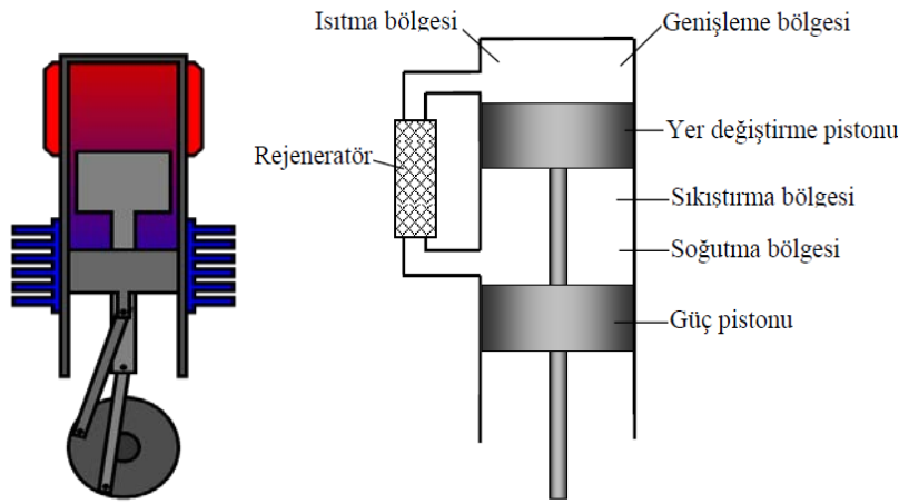
Şekil 3.6. Beta tipi Stirling motor prototipi ve displacer bloğu [20,35]
