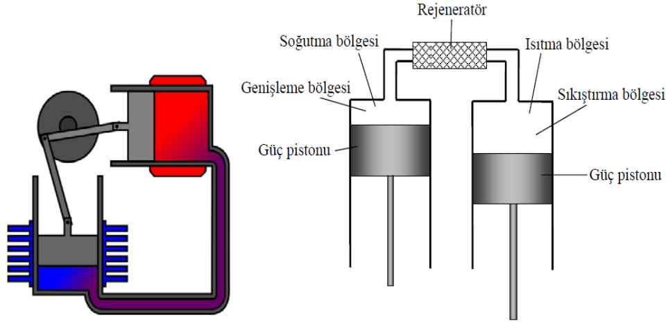
Şekil 3.5. Alfa tipi Stirling motor [20,35]
