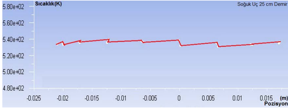
Şekil 4.14. 50 cm uzunluğundaki Demir displacer borusunun sıcaklık değişimi
