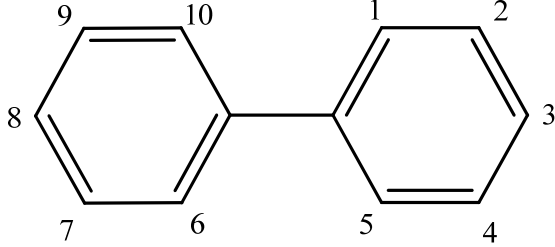
Şekil 4. Poliklorlubifenil.
