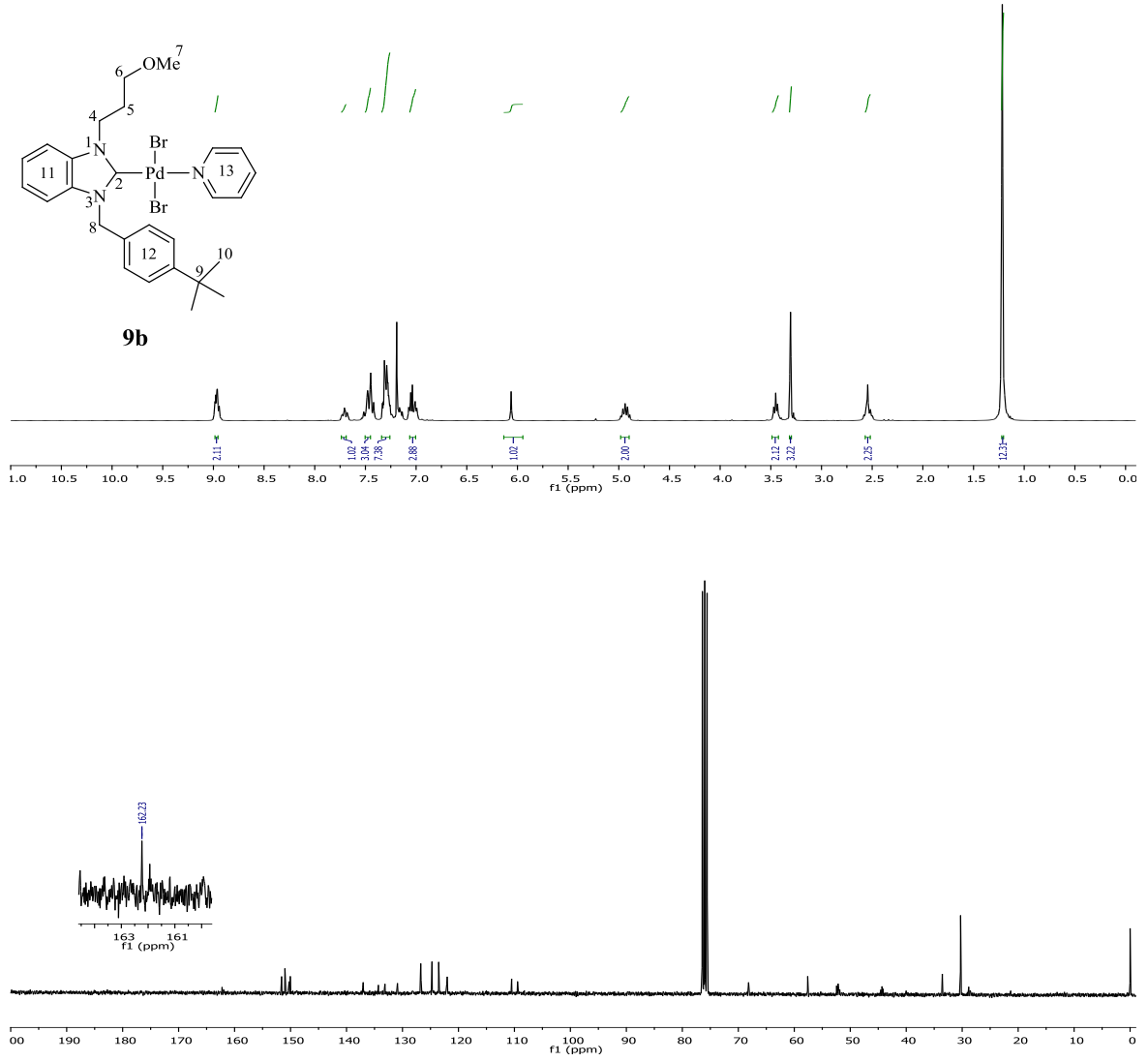
Şekil 3.44 9b Bileşiğine ait 1 H ve 13 C NMR spektrumları.
