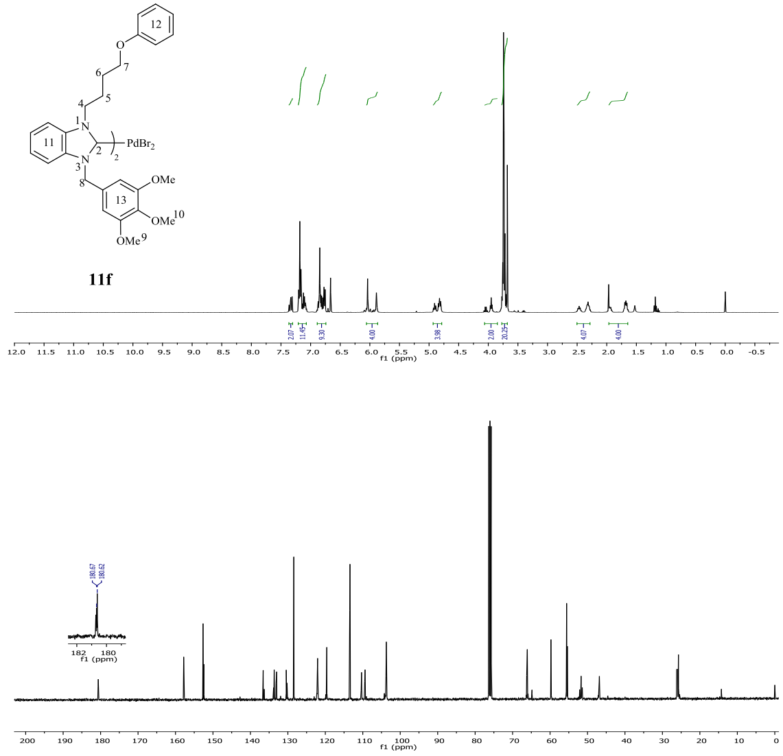
Şekil 3.62 11f Bileşiğine ait 1 H ve 13 C NMR spektrumları.
