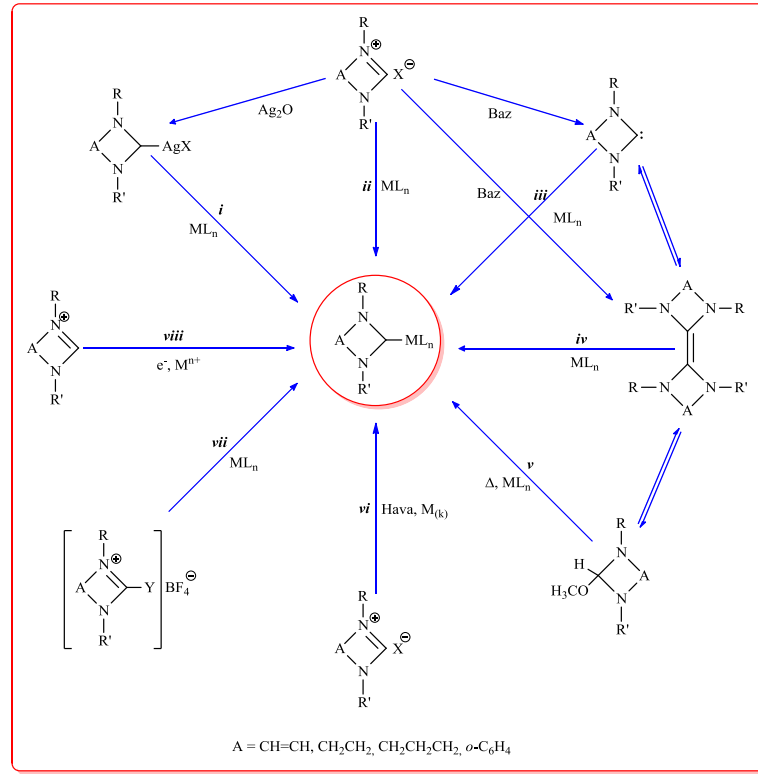
Şema 1.1 Metal-NHC komplekslerinin bazı sentez yöntemleri.
