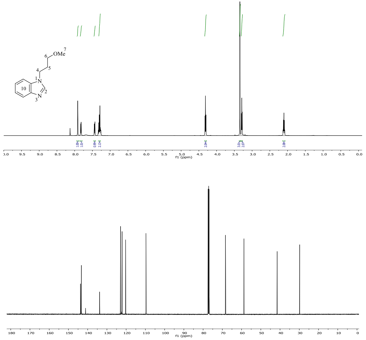
Şekil 3.7 N-(3-Metoksipropil)benzimidazol bileşiğine ait 1 H ve 13 C NMR spektrumları.
