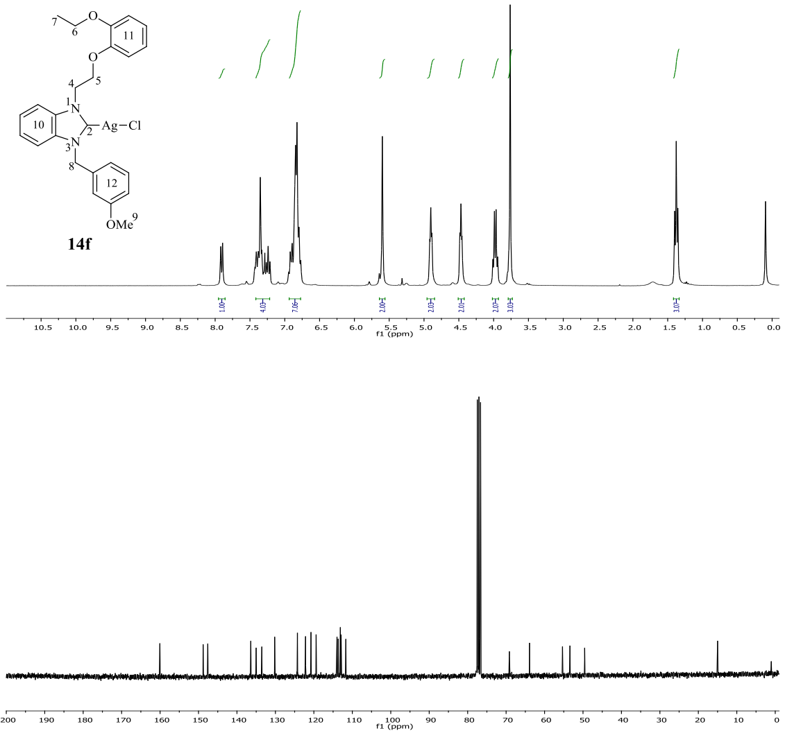
Şekil 3.81 14f Bileşiğine ait 1 H ve 13 C NMR spektrumları.
