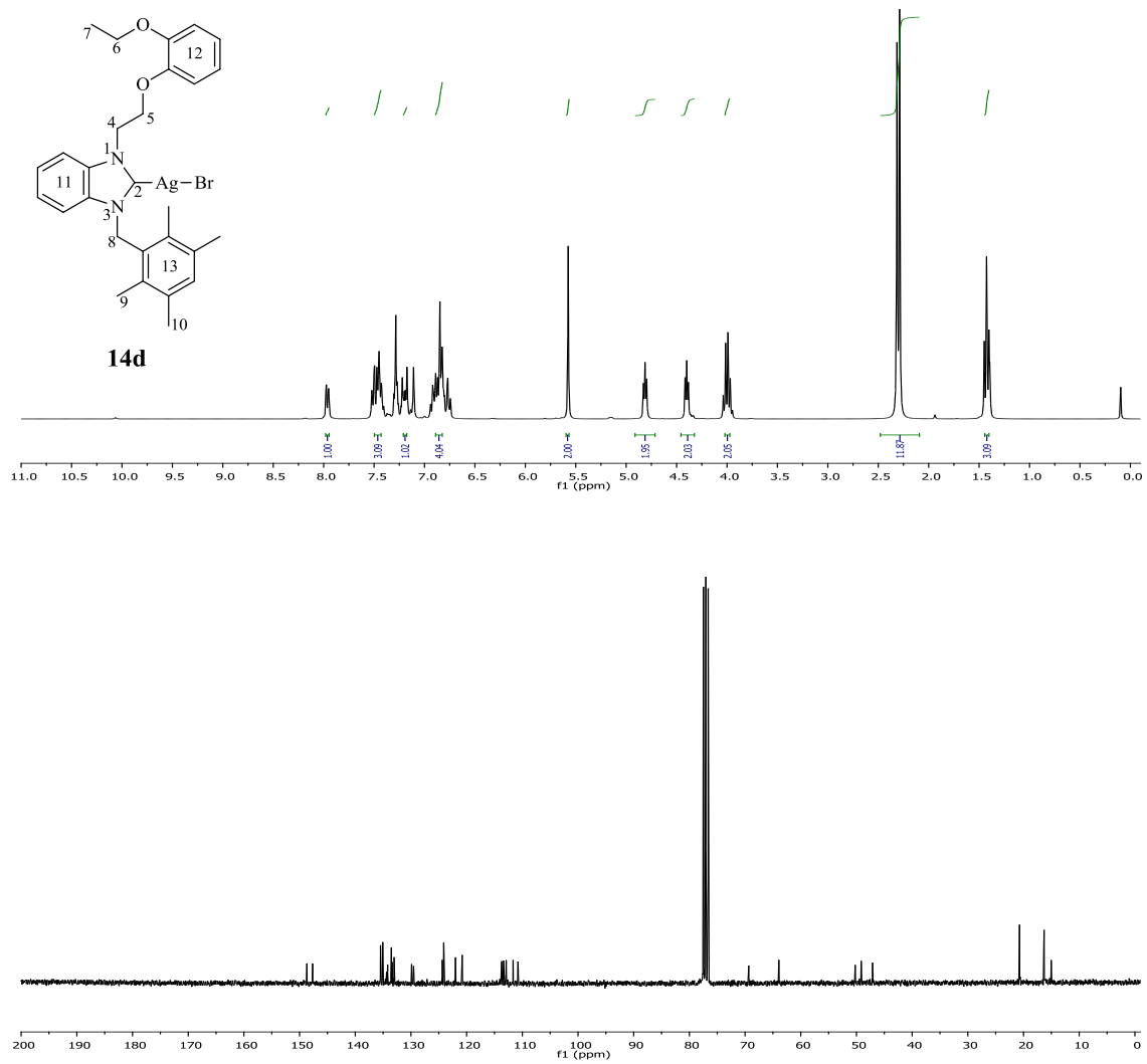
Şekil 3.79 14d Bileşiğine ait 1 H ve 13 C NMR spektrumları.
