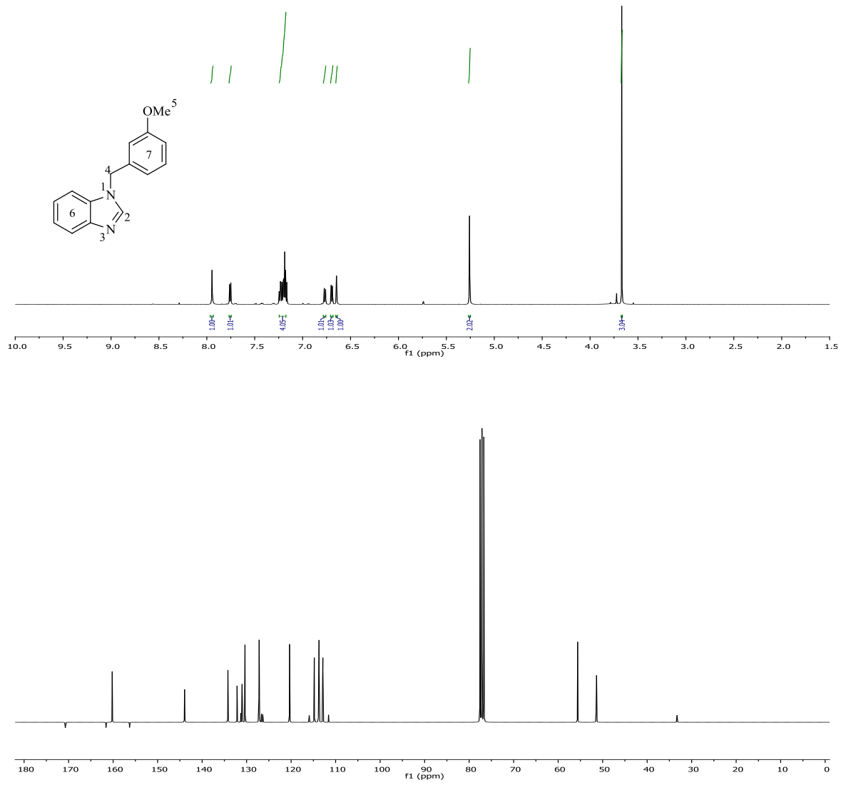
Şekil 3.25 N -(3-Metoksibenzil)benzimidazol bileşiğine ait 1 H ve 13 C NMR spektrumları
