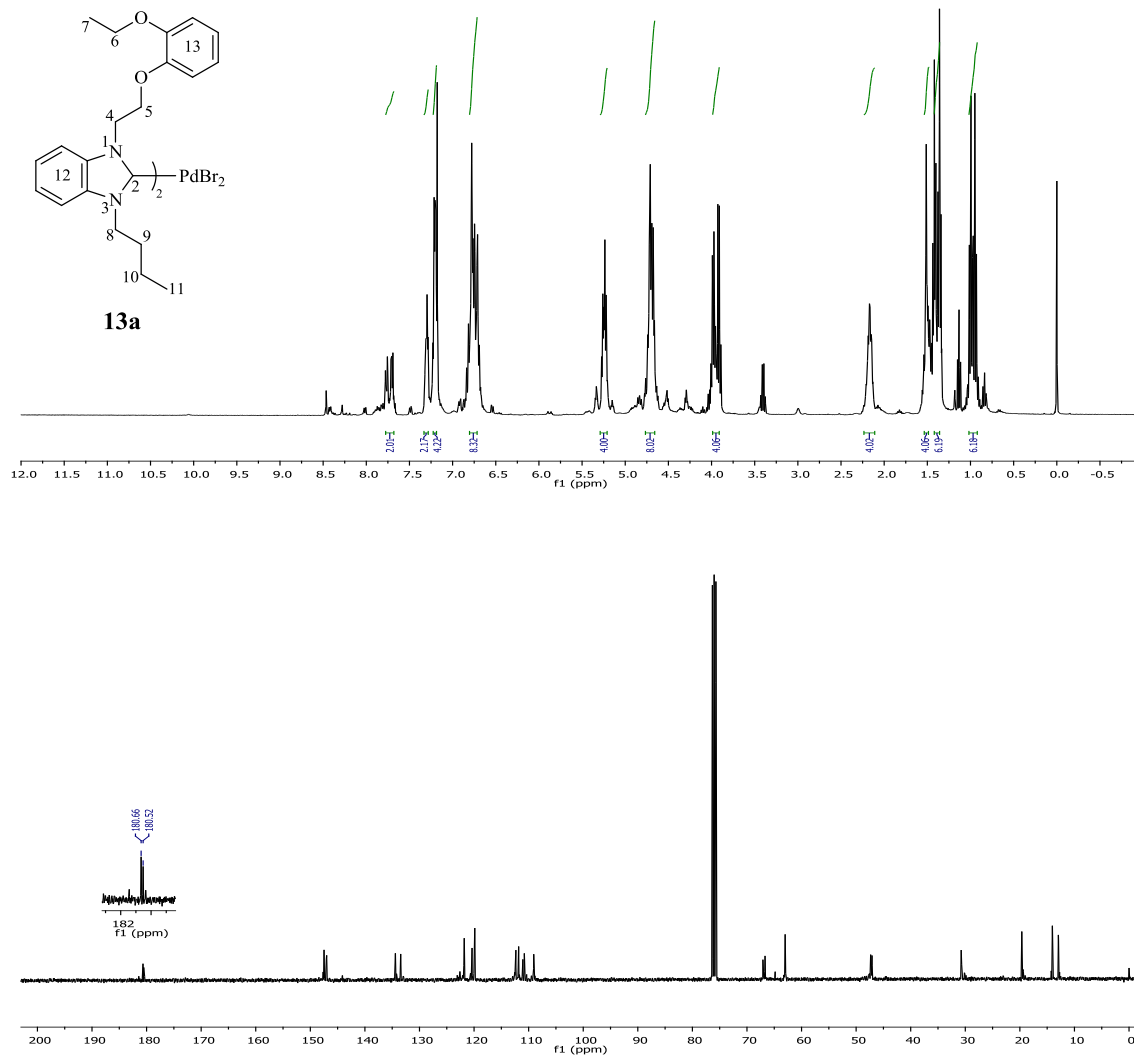
Şekil 3.70 13a Bileşiğine ait 1 H ve 13 C NMR spektrumları.
