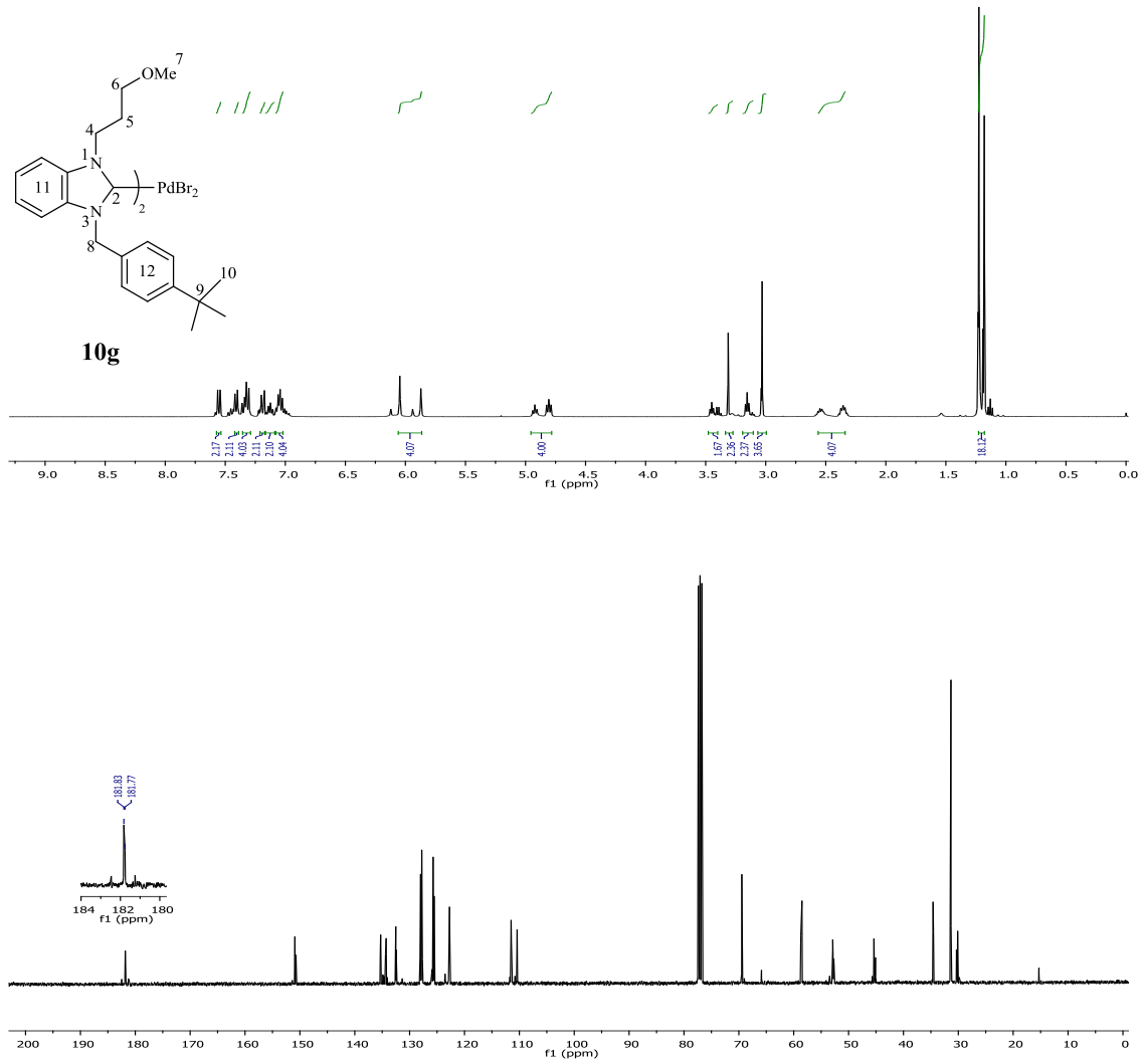
Şekil 3.56 10g Bileşiğine ait 1 H ve 13 C NMR spektrumları.
