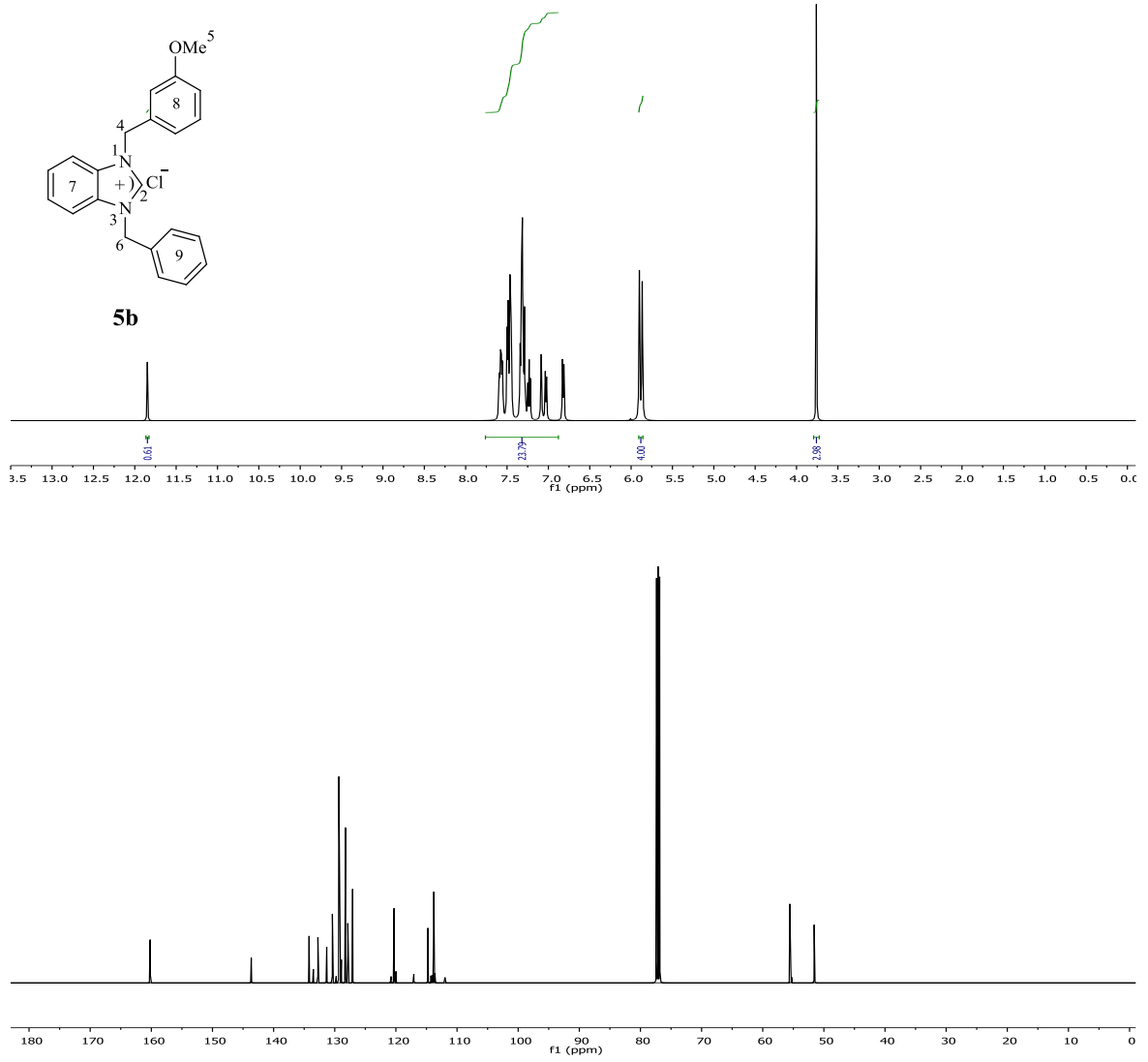
Şekil 3.27 5b Bileşiğine ait 1 H ve 13 C NMR spektrumları.
