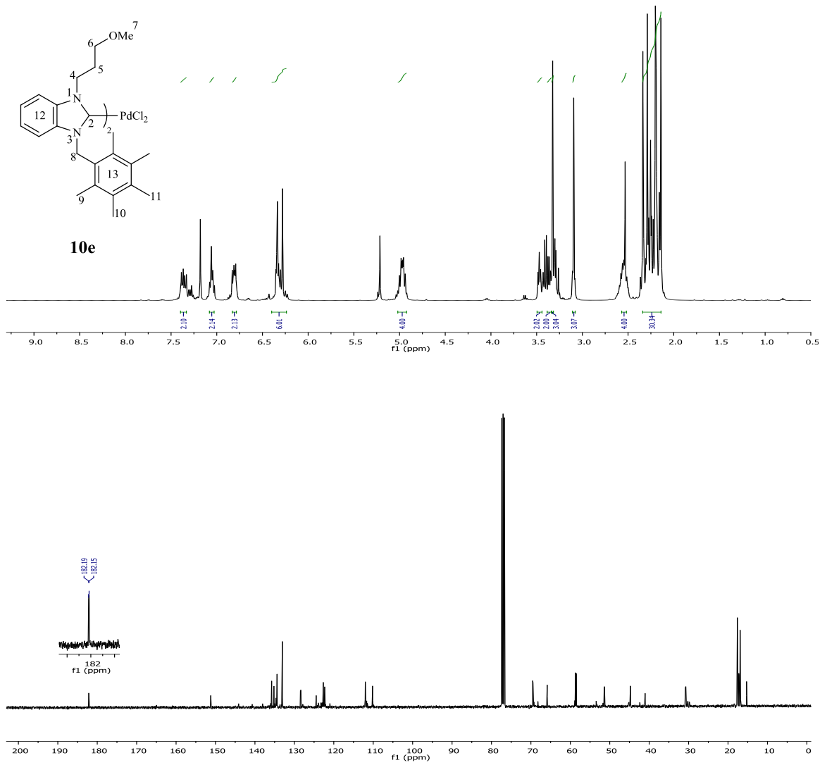
Şekil 3.54 10e Bileşiğine ait ^1\text{H} ve ^{13}\text{C} NMR spektrumları.
