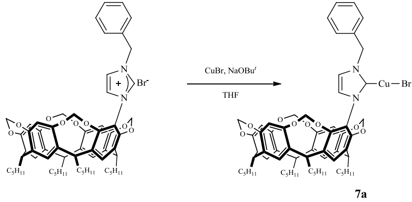
Şema 3.6 Sentezlenen resorsin[4]aren süstitüye Cu-NHC kompleksi.
