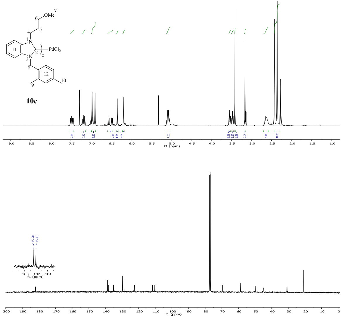
Şekil 3.52 10c Bileşiğine ait 1 H ve 13 C NMR spektrumları.
