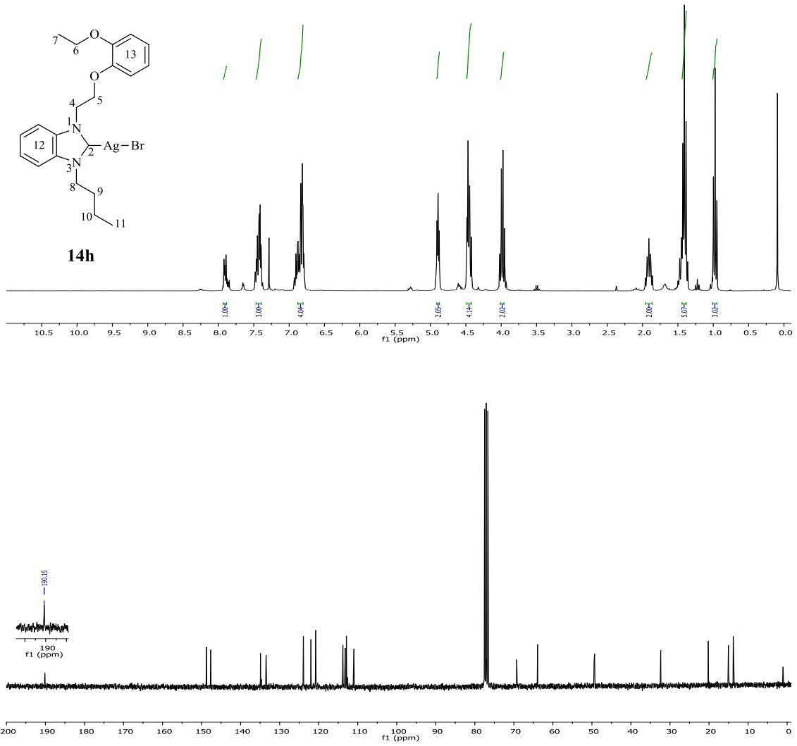
Şekil 3.83 14h Bileşiğine ait 1 H ve 13 C NMR spektrumları.
