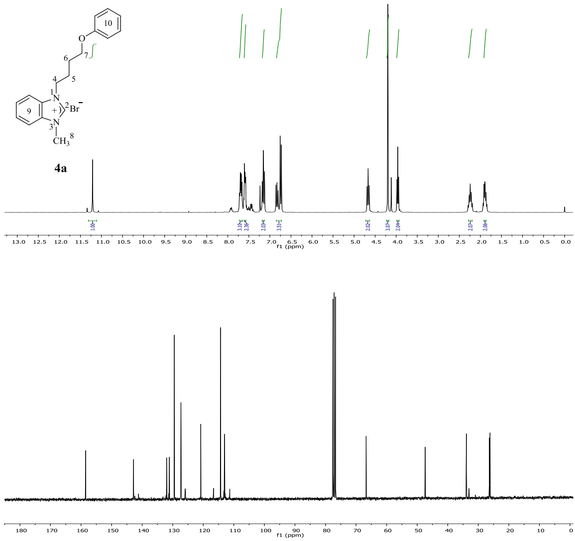
Şekil 3.18 4a Bileşiğine ait ^1\text{H} ve ^{13}\text{C} NMR spektrumları.
