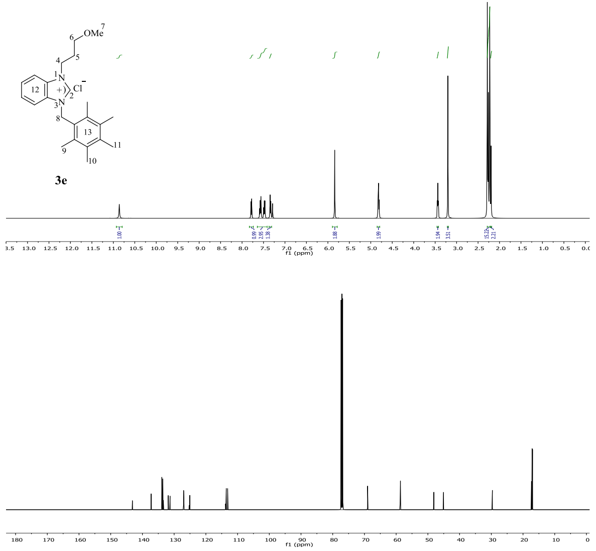
Şekil 3.12 3e Bileşiğine ait 1 H ve 13 C NMR spektrumları.
