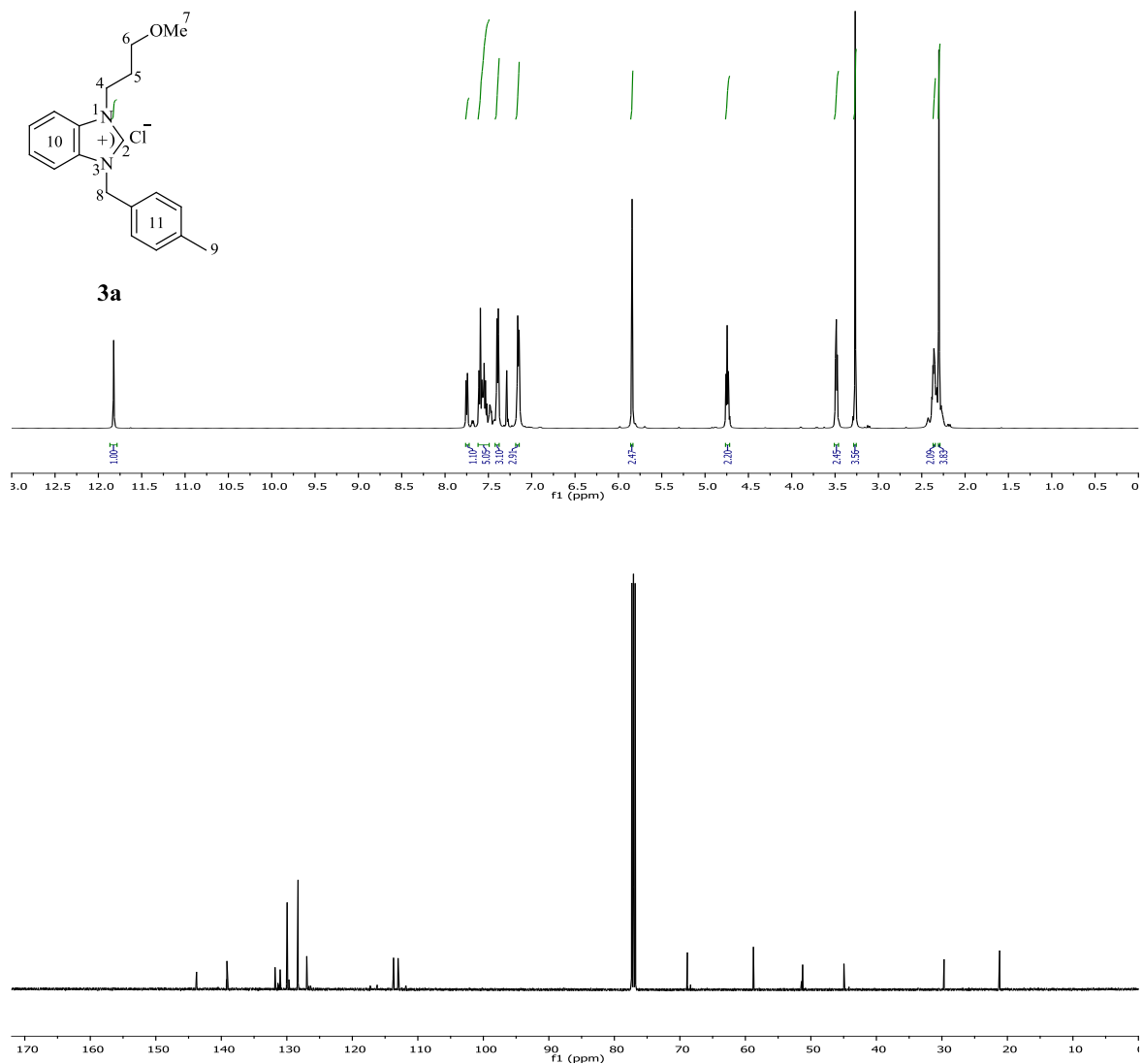
Şekil 3.8 3a Bileşiğine ait 1 H ve 13 C NMR spektrumları.
