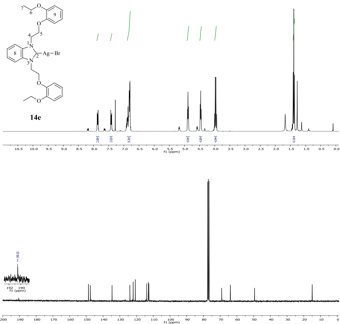
Şekil 3.80 14e Bileşiğine ait 1 H ve 13 C NMR spektrumları.
