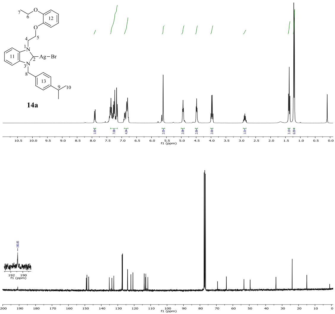
Şekil 3.76 14a Bileşiğine ait ^1\text{H} ve ^{13}\text{C} NMR spektrumları.
