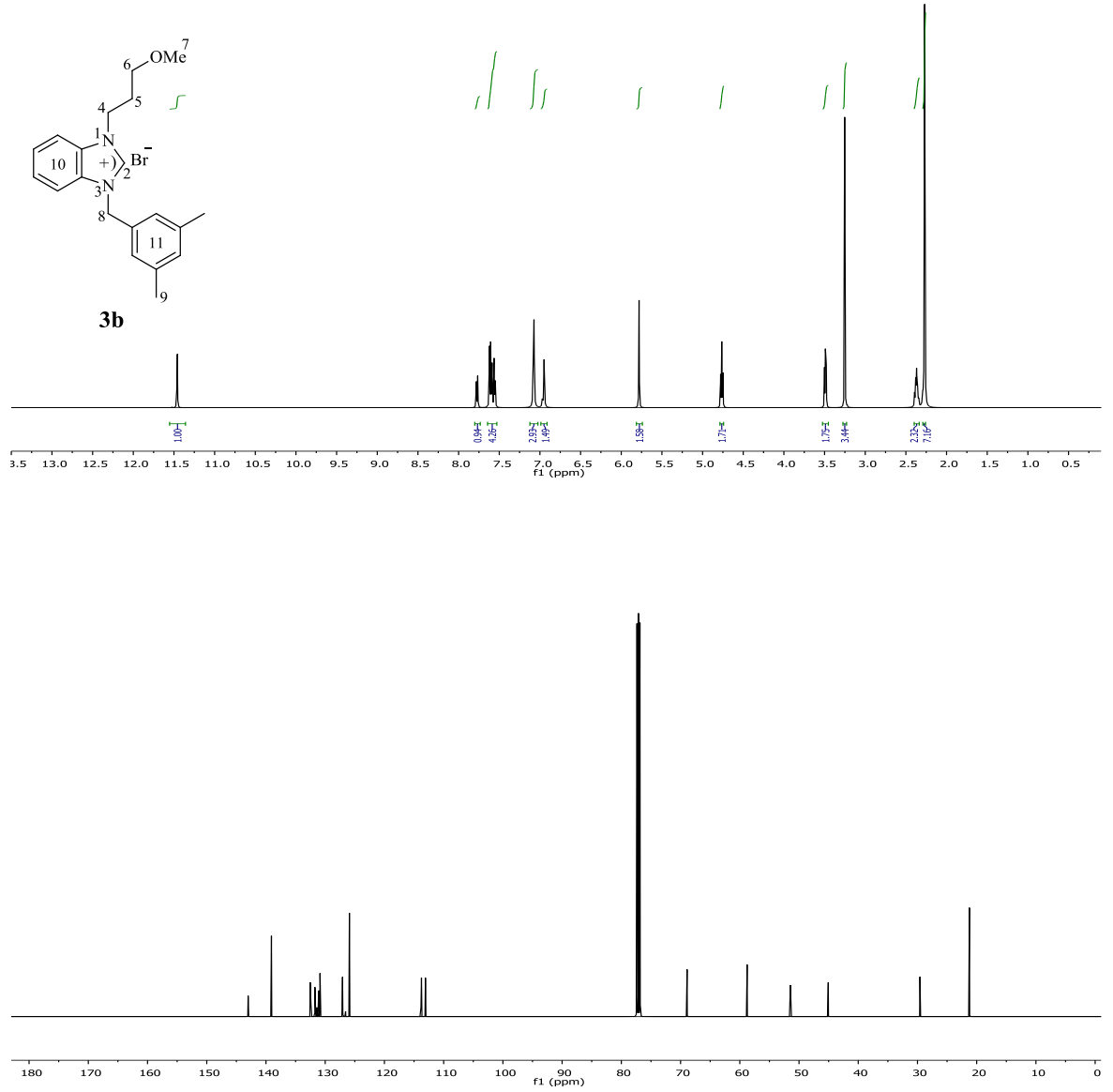
Şekil 3.9 3b Bileşiğine ait 1 H ve 13 C NMR spektrumları.
