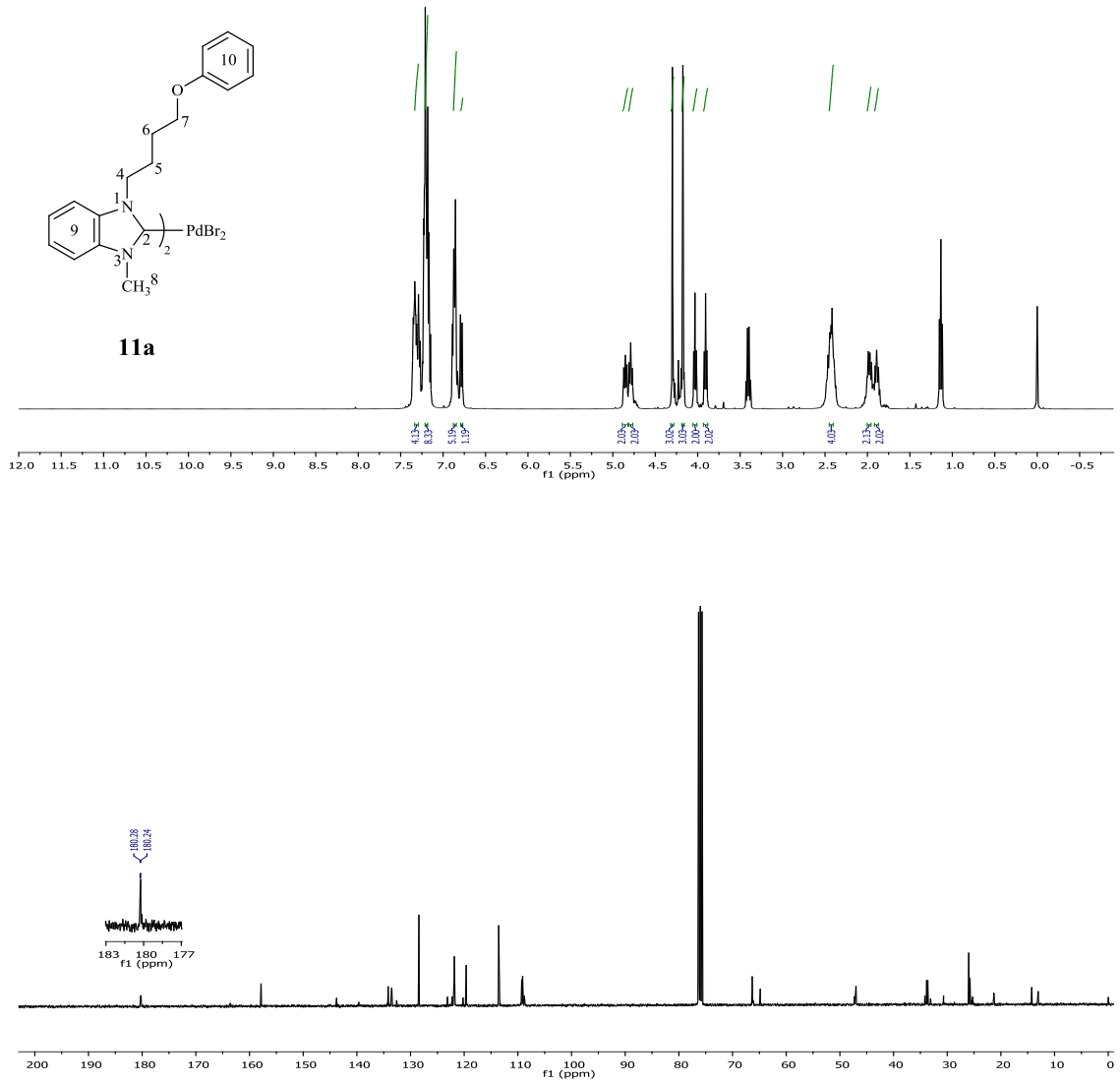
Şekil 3.57 11a Bileşiğine ait 1 H ve 13 C NMR spektrumları.
