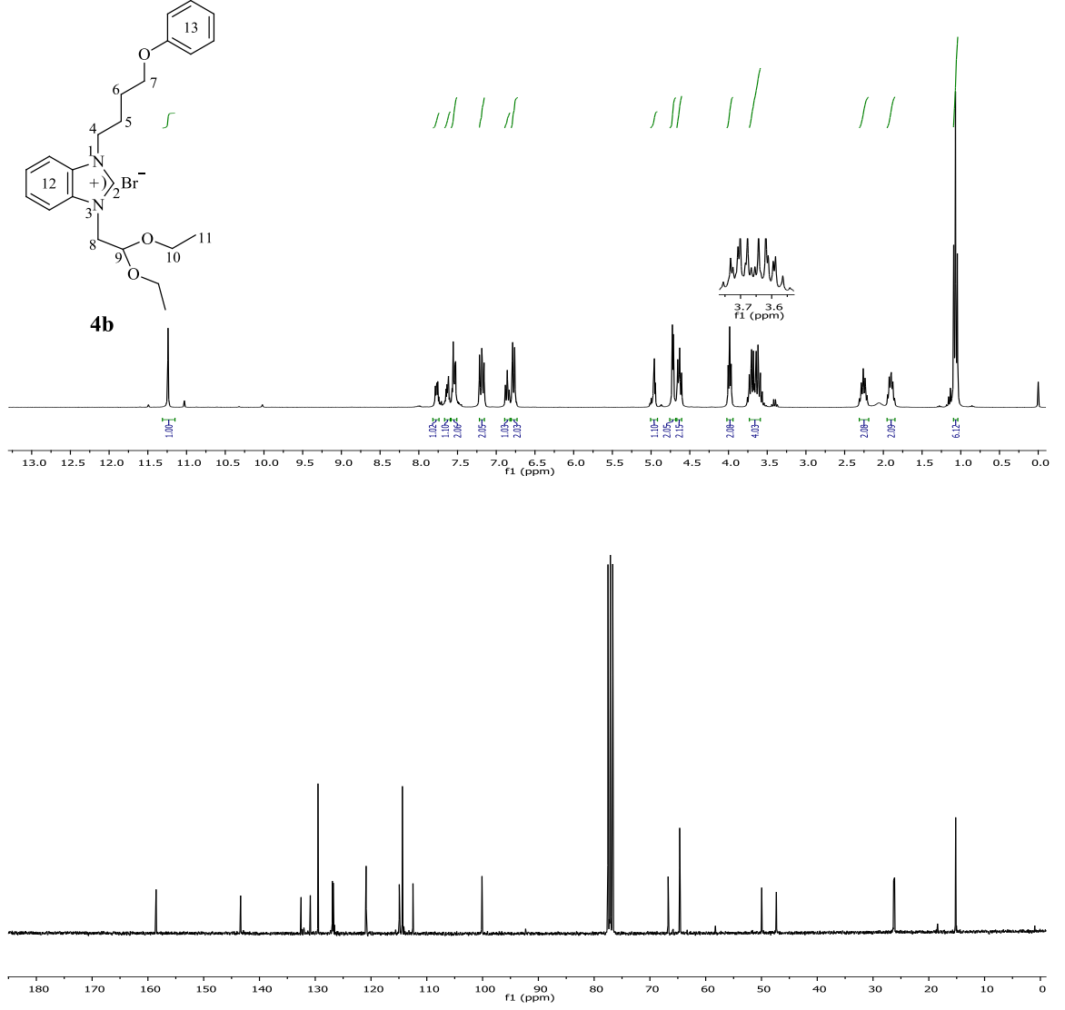
Şekil 3.19 4b Bileşiğine ait ^1\text{H} ve ^{13}\text{C} NMR spektrumları.
