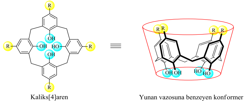
Şekil 1.14 Tetramer yapıdaki kaliks[4]aren halkasının yapısı ve Yunan vazosuna benzeyen konformeri.
