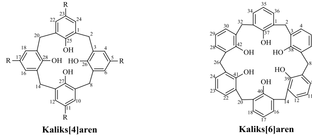
Şekil 1.19 Kaliks[n]aren halkalarının numaralandırılması.
