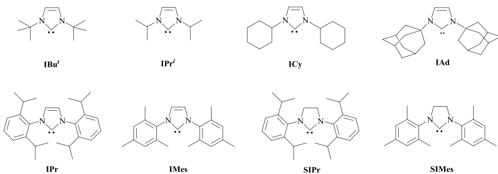
Şekil 1.5 Ticari öneme sahip bazı imidazol-2-iliden ve imidazolidin-2-iliden ligandları.
