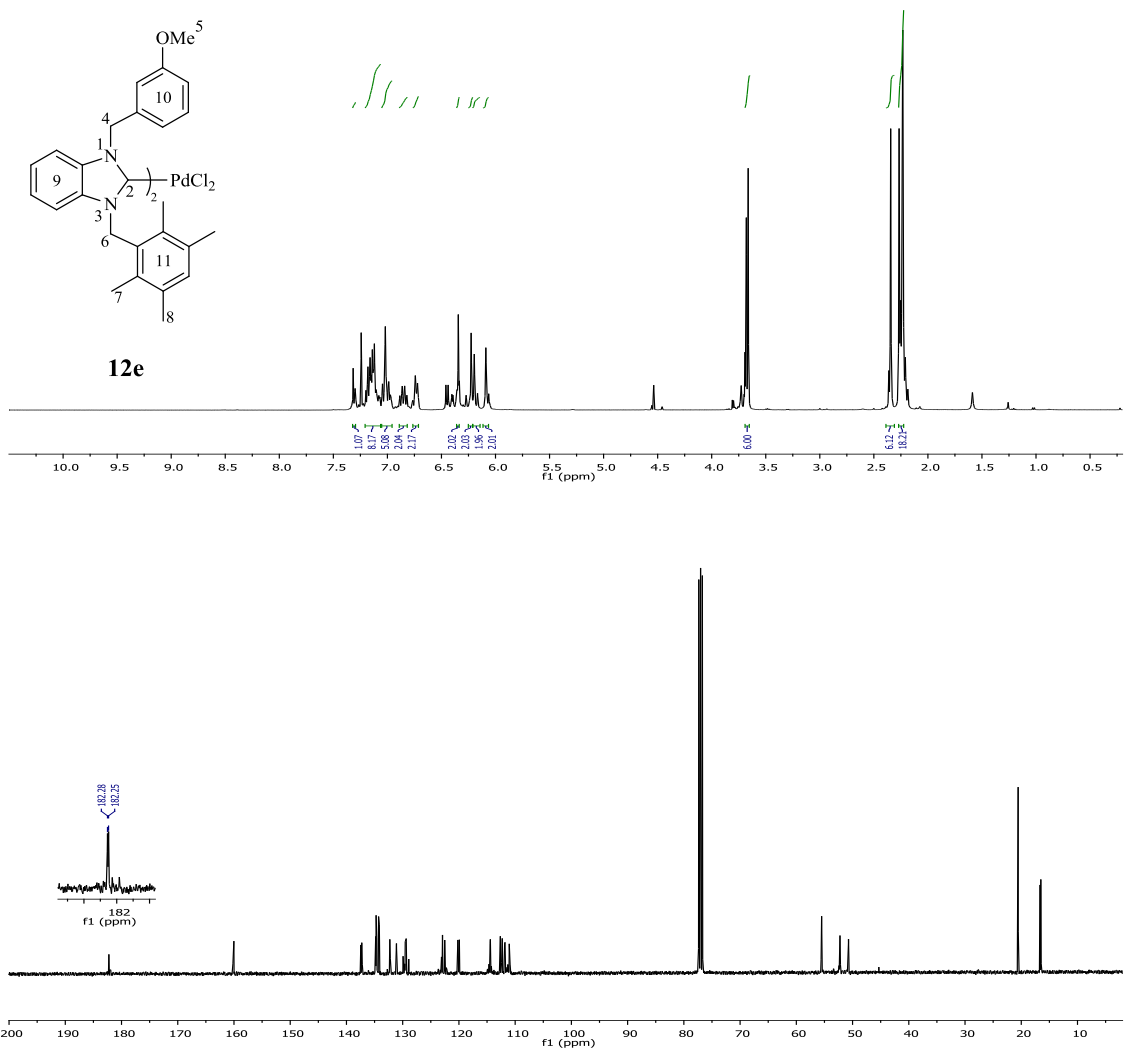
Şekil 3.68 12e Bileşiğine ait 1 H ve 13 C NMR spektrumları.
