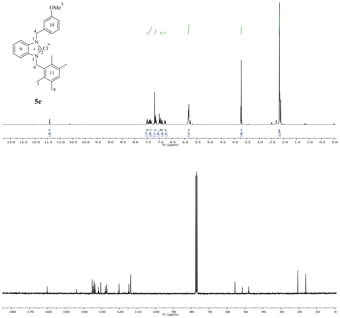
Şekil 3.30 5e Bileşiğine ait ^1\text{H} ve ^{13}\text{C} NMR spektrumları.
