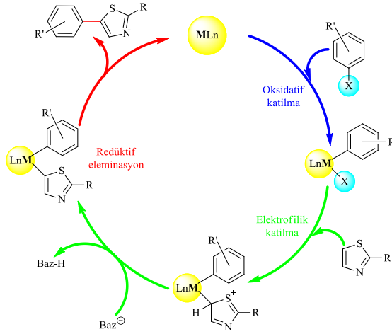
Şema 1.6 Aril halojenürlerin kullanıldığı direkt arilasyon tepkimelerine ait katalitik çevrim.
