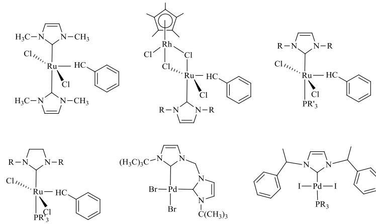
Şekil 1.13 Olefin metatezinde kullanılan bazı Ru-NHC ve Pd-NHC kompleksleri.
