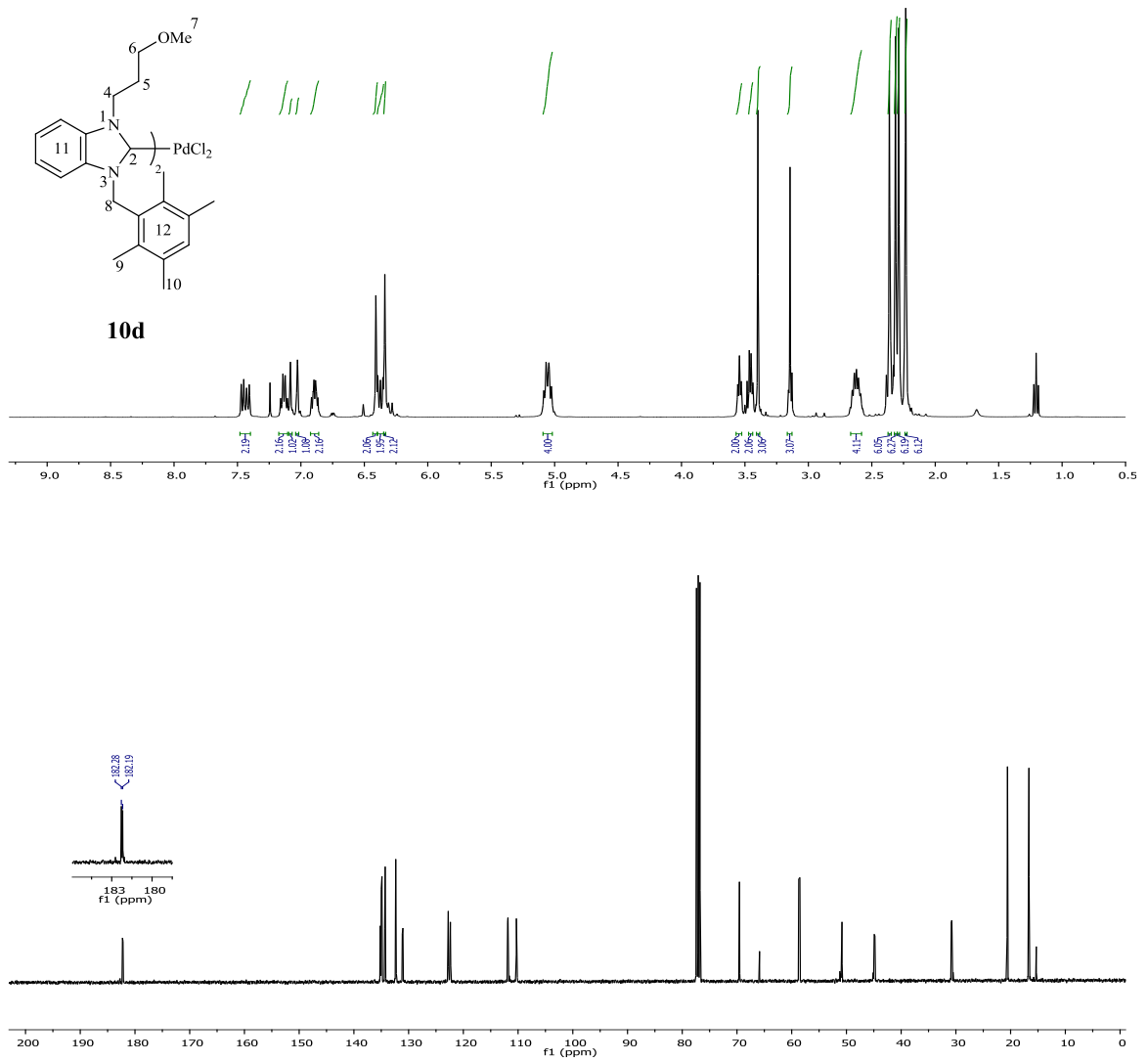
Şekil 3.53 10d Bileşiğine ait 1 H ve 13 C NMR spektrumları.
