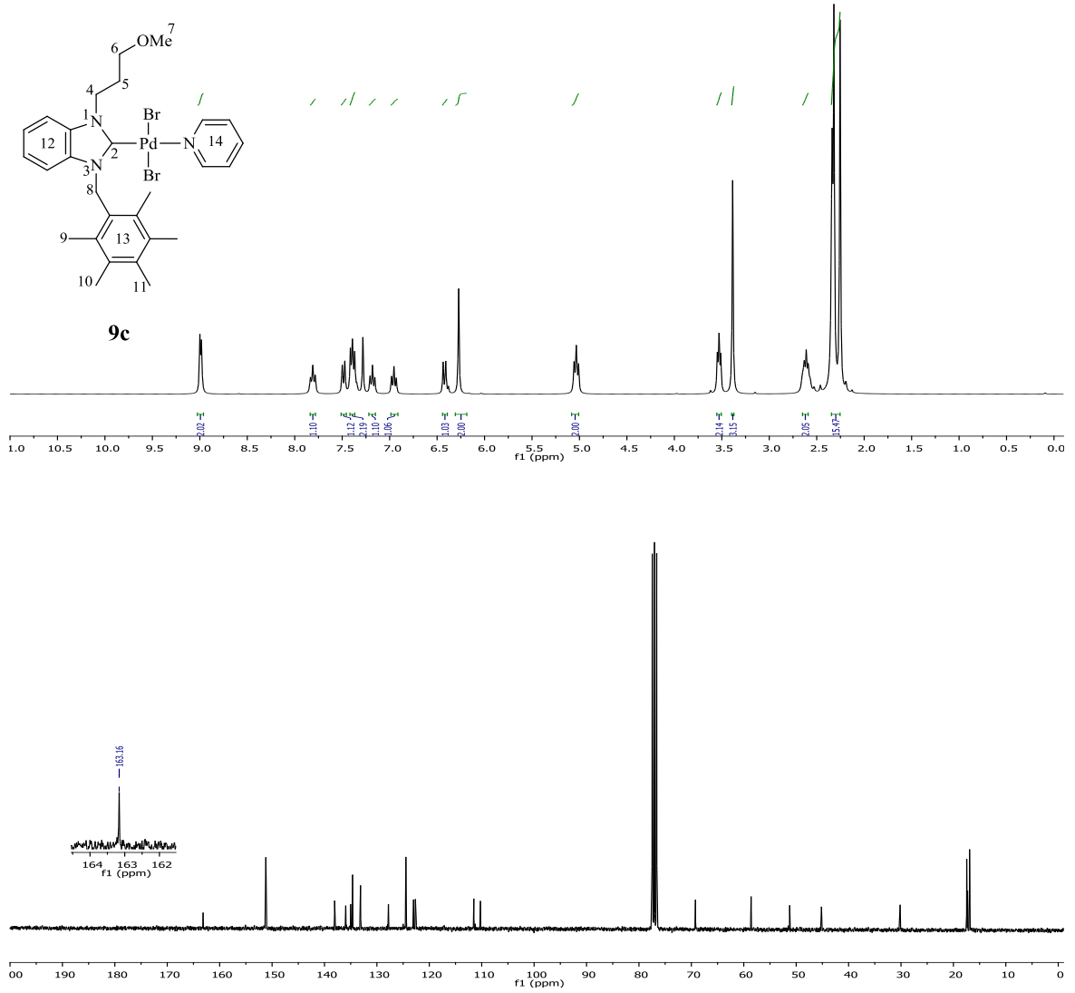
Şekil 3.45 9c Bileşiğine ait 1 H ve 13 C NMR spektrumları.
