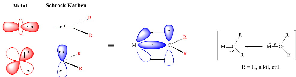
Şekil 1.9 Schrock tipi karben komplekslerinde bağlanma ve rezonans yapıları.
