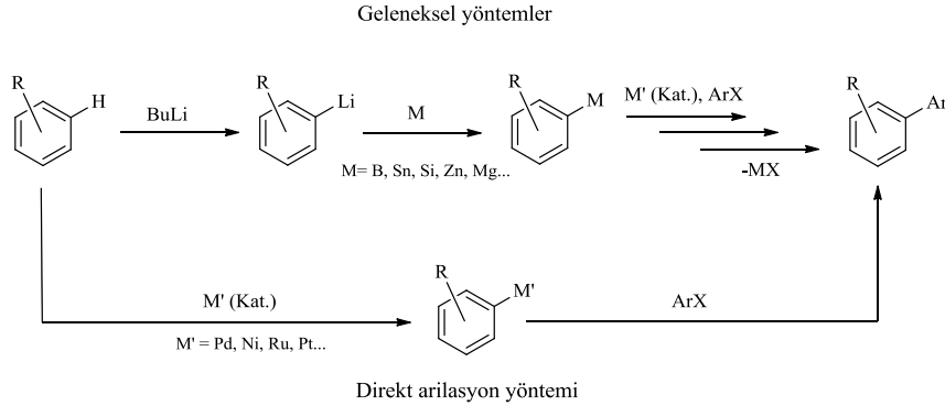
Şema 1.4 Geleneksel yöntemler ve direkt arilasyon yönteminin karşılaştırılması.
