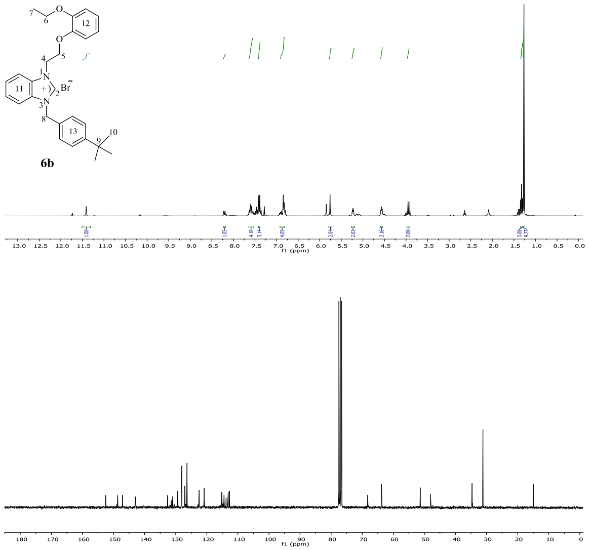
Şekil 3.33 6b Bileşiğine ait 1 H ve 13 C NMR spektrumları.
