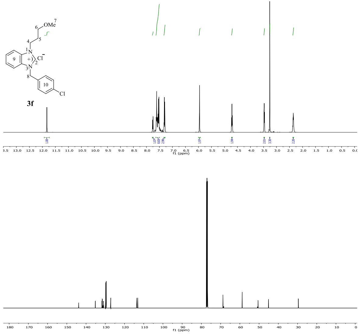
Şekil 3.13 3f Bileşiğine ait 1 H ve 13 C NMR spektrumları.
