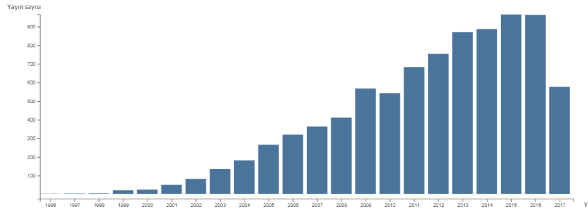
Şekil 1.7 NHC'ler ile ilgili yayınlanmış çalışmaların yıllara göre dağılımı (*).
