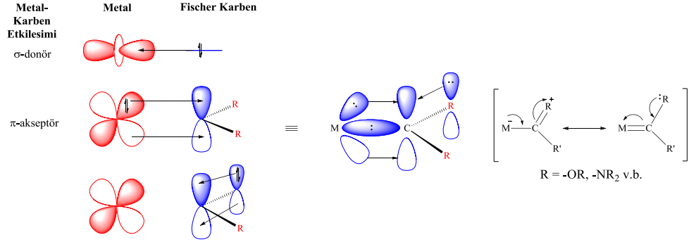
Şekil 1.8 Fischer tipi karben komplekslerinde bağlanma ve rezonans yapıları.
