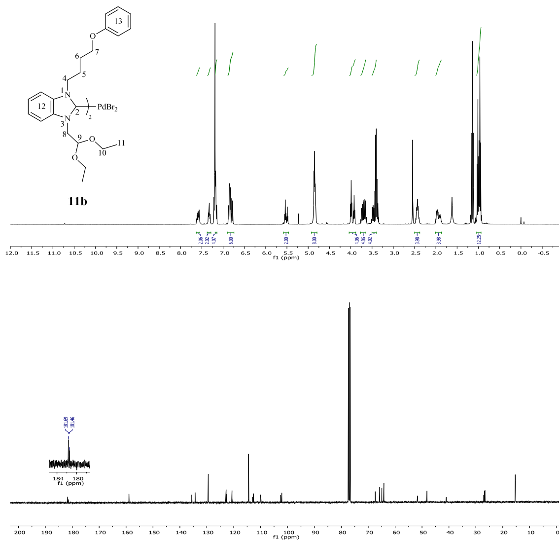
Şekil 3.58 11b Bileşiğine ait 1 H ve 13 C NMR spektrumları.
