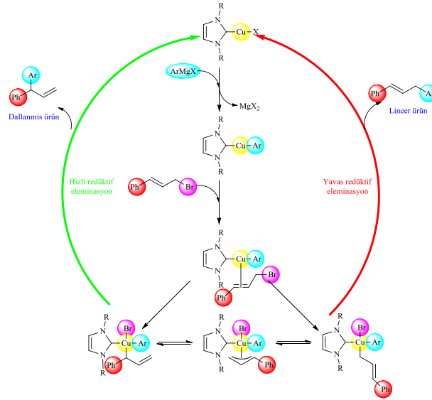
Şema 1.7 Sınnamil bromürün Grignard bileşikleri ile bakır katalizli allilik sübstütüsyonuna ait katalitik çevrim.
