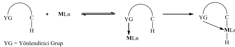
Şema 1.5 Yönlendirici grubun C-H bağının rejioseçici moleküliçi ayrılmasındaki rolü.
