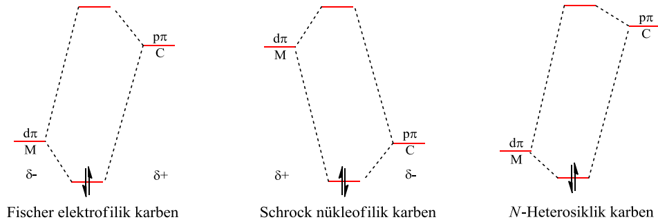
Şekil 1.11 Fischer, Schrock ve NHC komplekslerinde enerji farkları.
