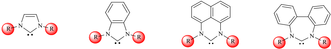
Şekil 1.2 Farklı halka büyüklüğüne sahip bazı NHC'ler.
