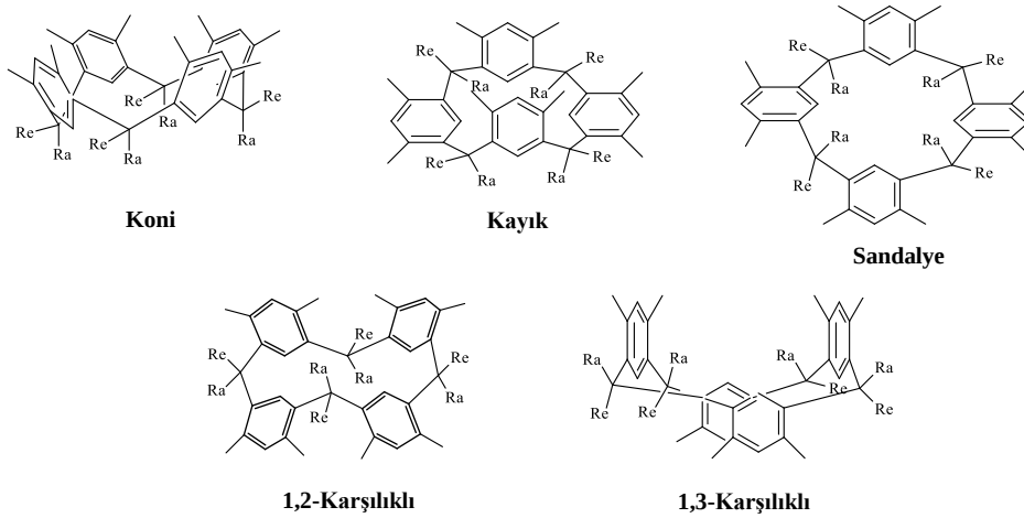
Şekil 1.17 Tetramerik yapıdaki resorsin[4]aren halkasına ait konformasyonlar.
