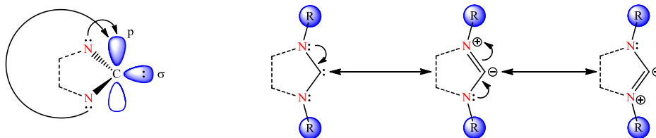
Şekil 1.3 Azottaki elektron çiftinin \pi -bağı yoluyla karben karbonuna aktarılması.
