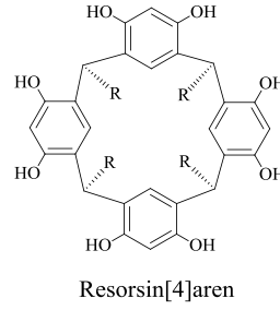
Şekil 1.16 Tetramerik yapılı resorsin[4]aren halkasının genel gösterimi.
