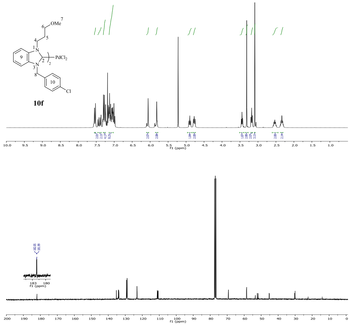
Şekil 3.55 10f Bileşiğine ait 1 H ve 13 C NMR spektrumları.
