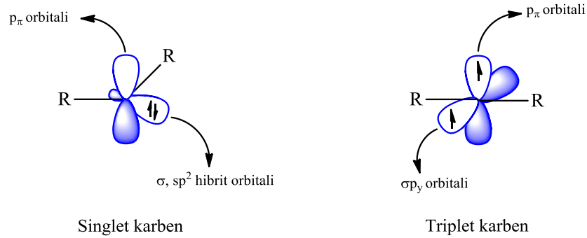
Şekil 1.1 Singlet ve triplet karbenlerin elektronik konfigürasyonları.
