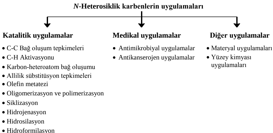
Şema 1.2 N-Heterosiklik karbenlerin uygulama alanları.
