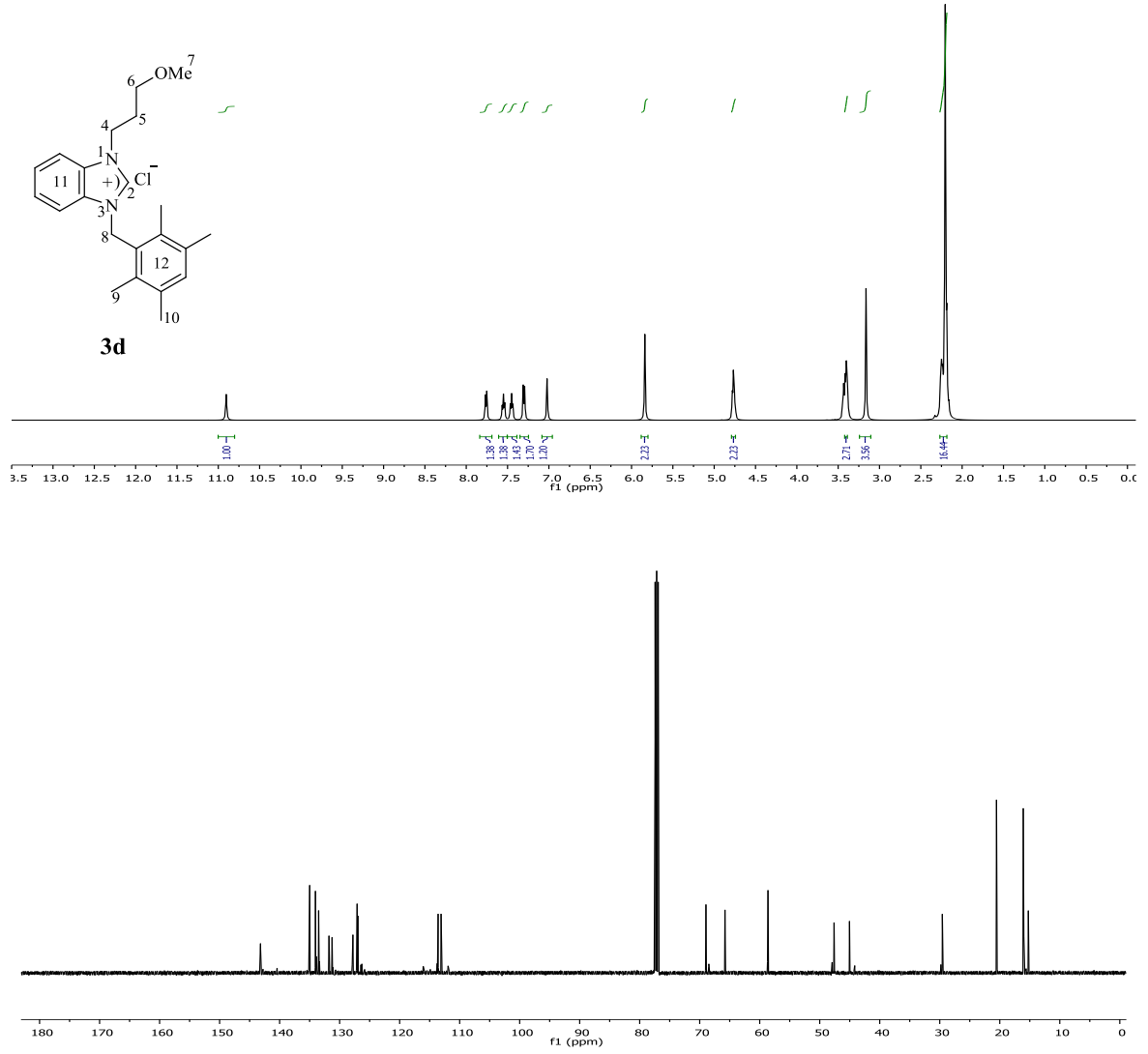
Şekil 3.11 3d Bileşiğine ait 1 H ve 13 C NMR spektrumları.
