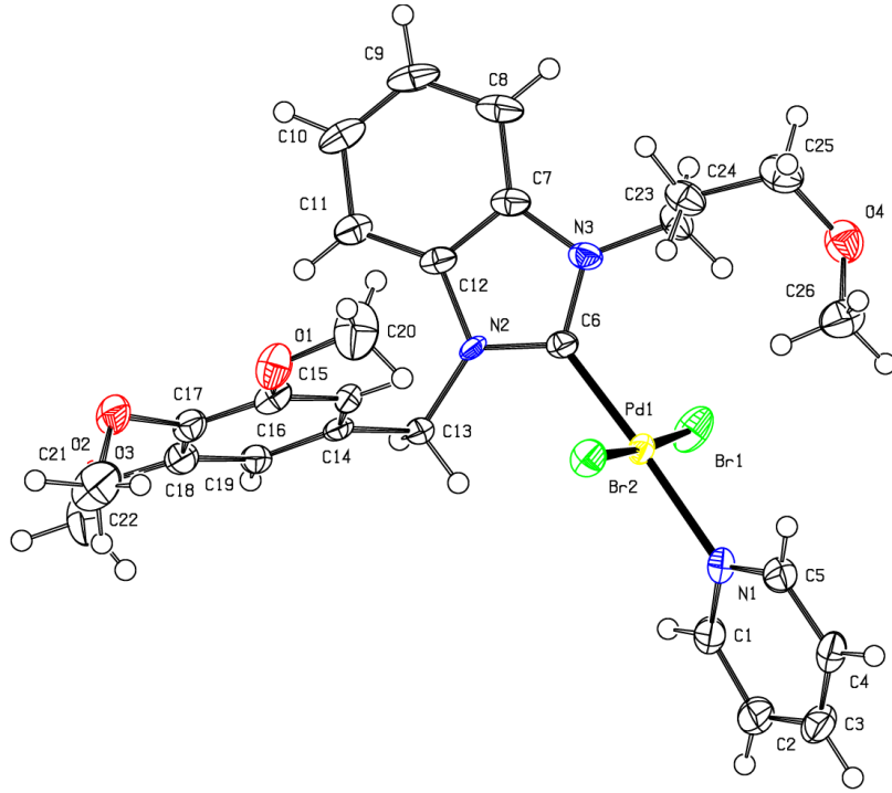
Şekil 3.49 9f Bileşiğinin X-ışını yapısı.
