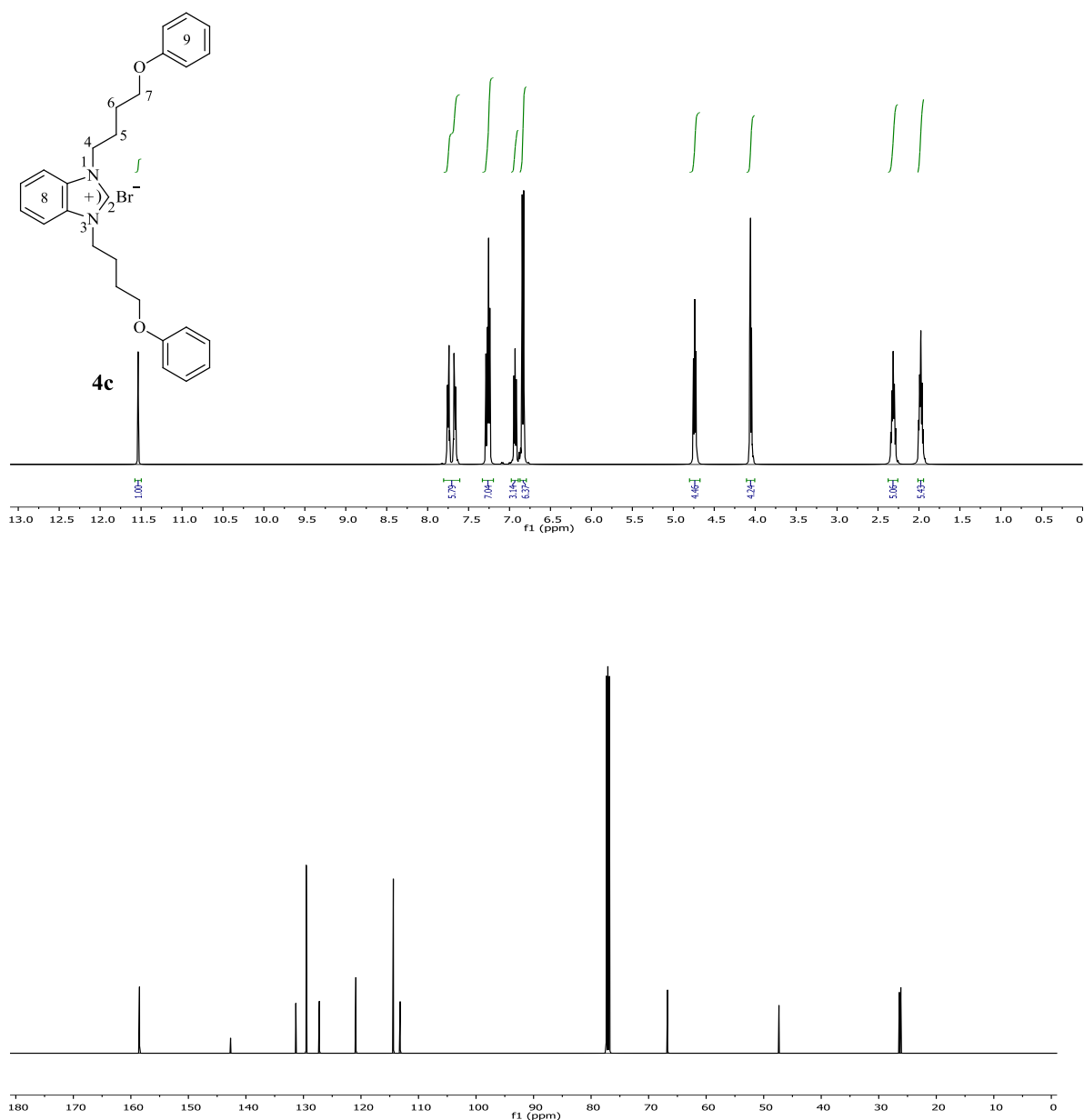
Şekil 3.20 4c Bileşiğine ait 1 H ve 13 C NMR spektrumları.
