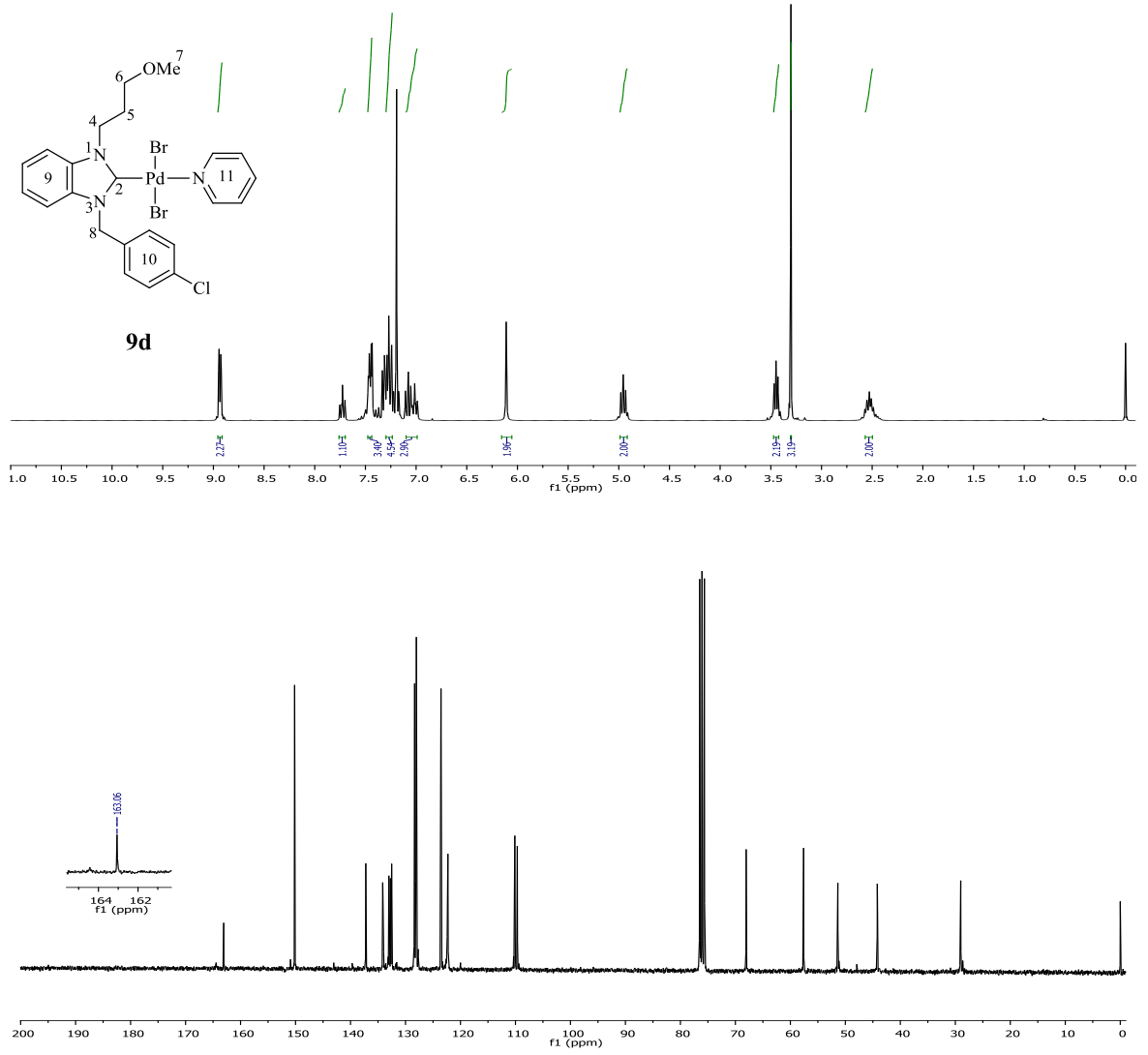
Şekil 3.46 9d Bileşiğine ait 1 H ve 13 C NMR spektrumları.
