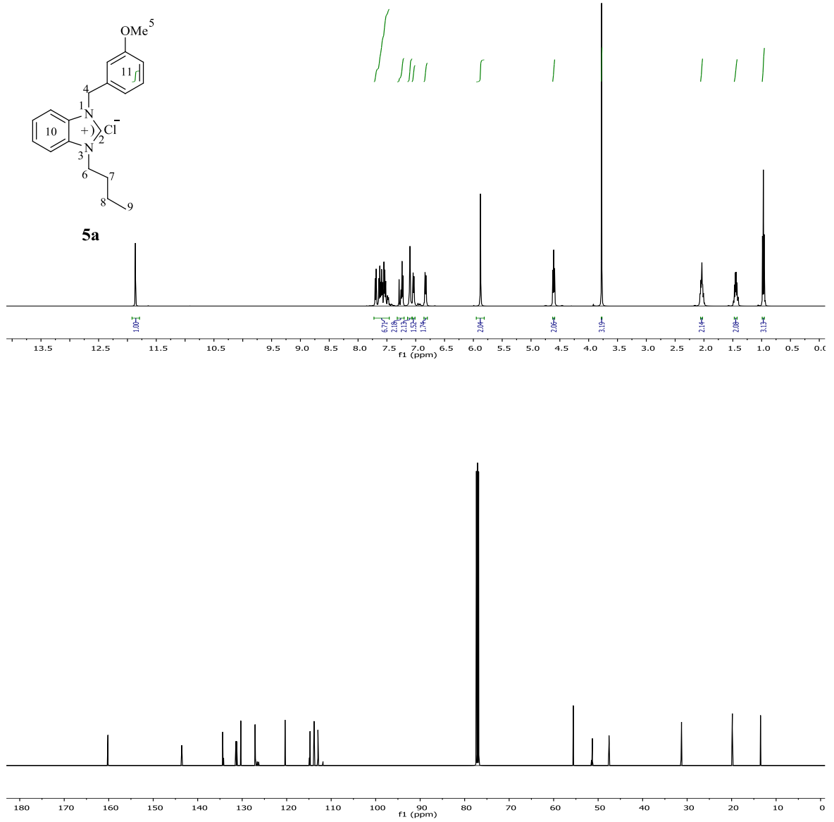
Şekil 3.26 5a Bileşiğine ait 1 H ve 13 C NMR spektrumları.
