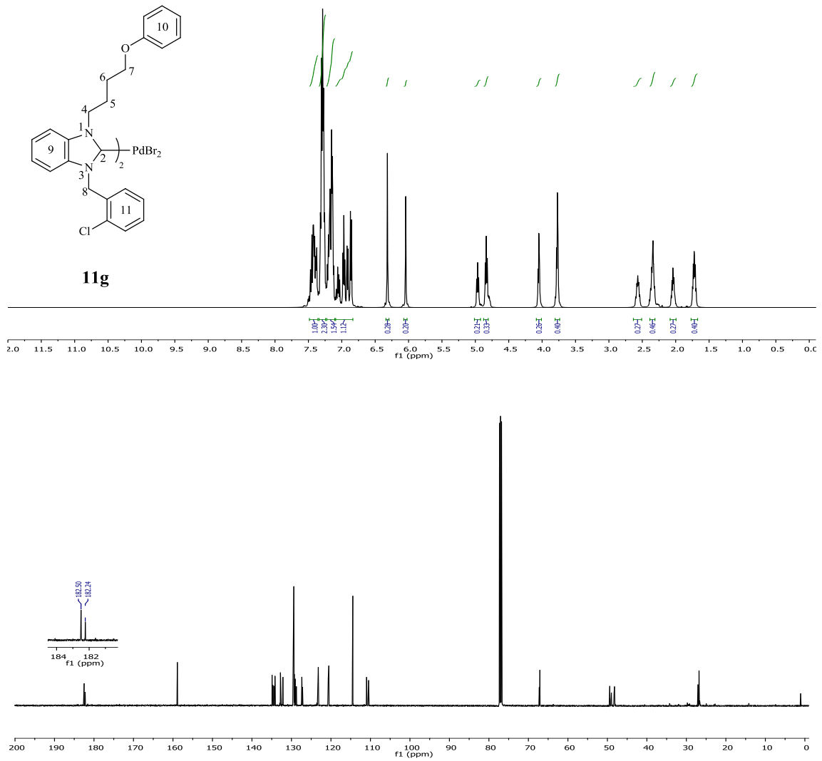
Şekil 3.63 11g Bileşiğine ait 1 H ve 13 C NMR spektrumları.
