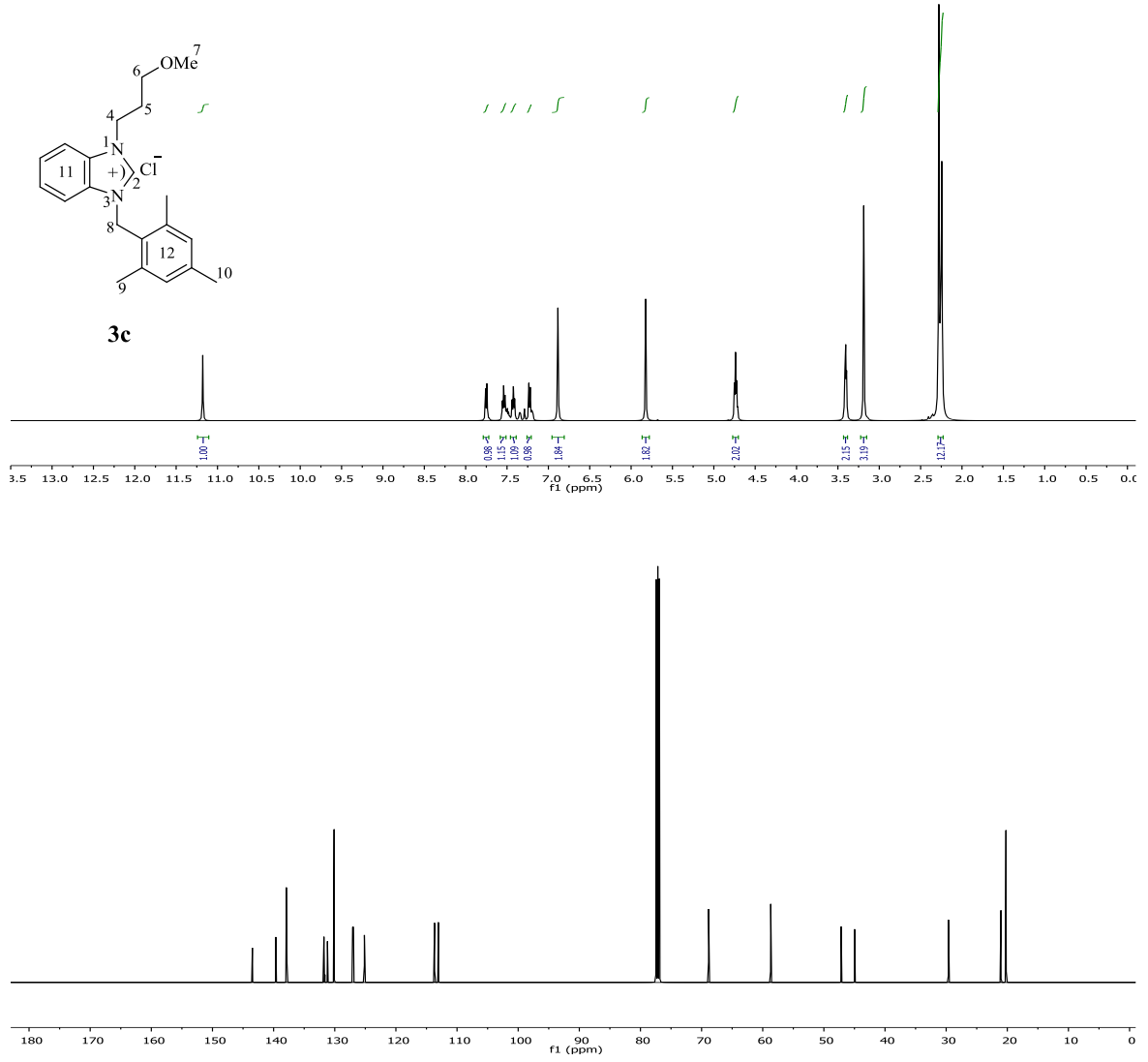
Şekil 3.10 3c Bileşiğine ait 1 H ve 13 C NMR spektrumları.
