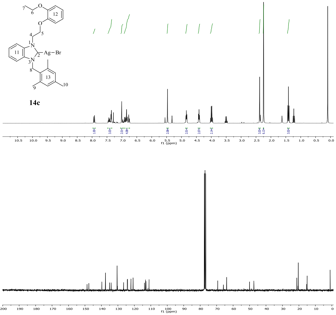
Şekil 3.78 14c Bileşiğine ait 1 H ve 13 C NMR spektrumları.
