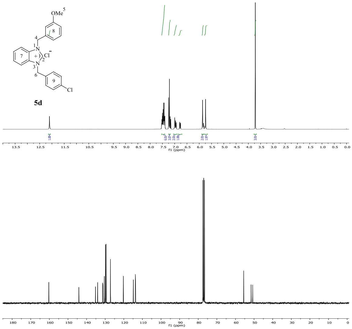
Şekil 3.29 5d Bileşiğine ait 1 H ve 13 C NMR spektrumları.
