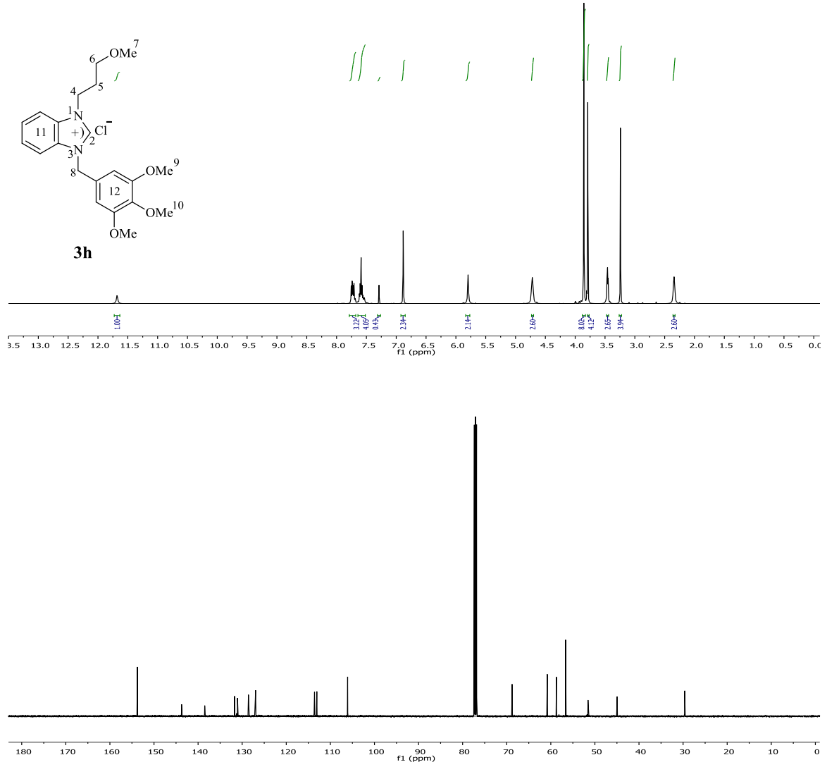
Şekil 3.15 3h Bileşiğine ait 1 H ve 13 C NMR spektrumları.
