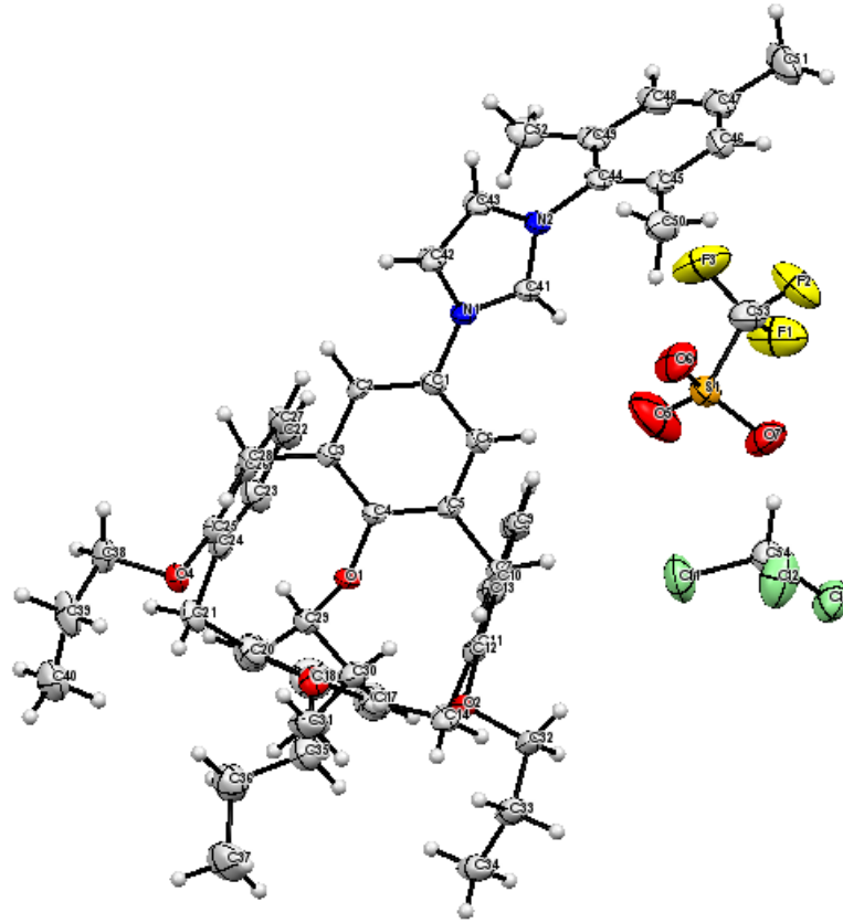
Şekil 3.4 1b Bileşiğinin X-ışını yapısı.
