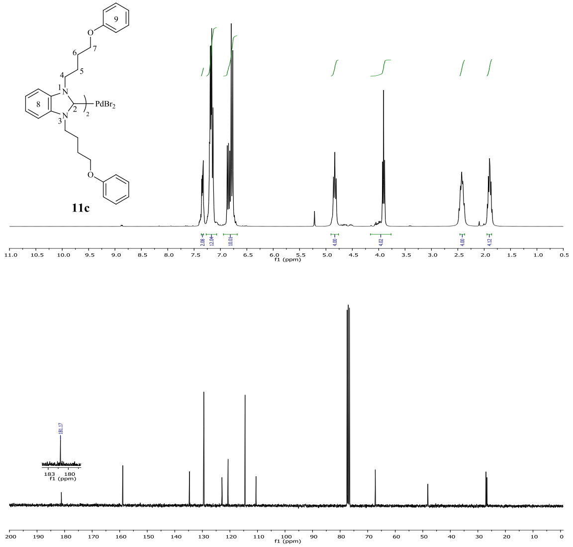
Şekil 3.59 11c Bileşiğine ait 1 H ve 13 C NMR spektrumları.
