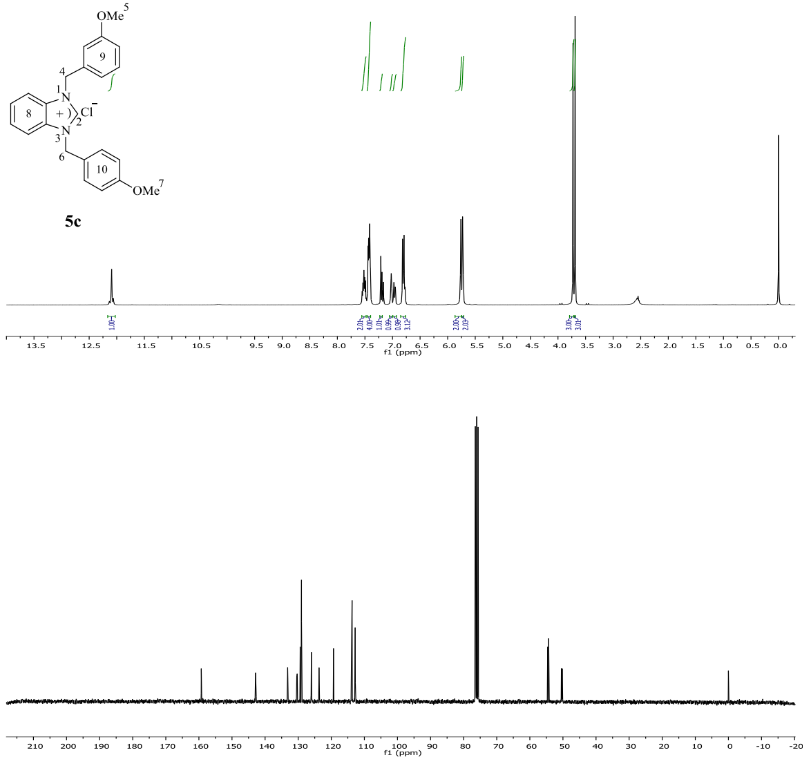
Şekil 3.28 5c Bileşiğine ait 1 H ve 13 C NMR spektrumları.
