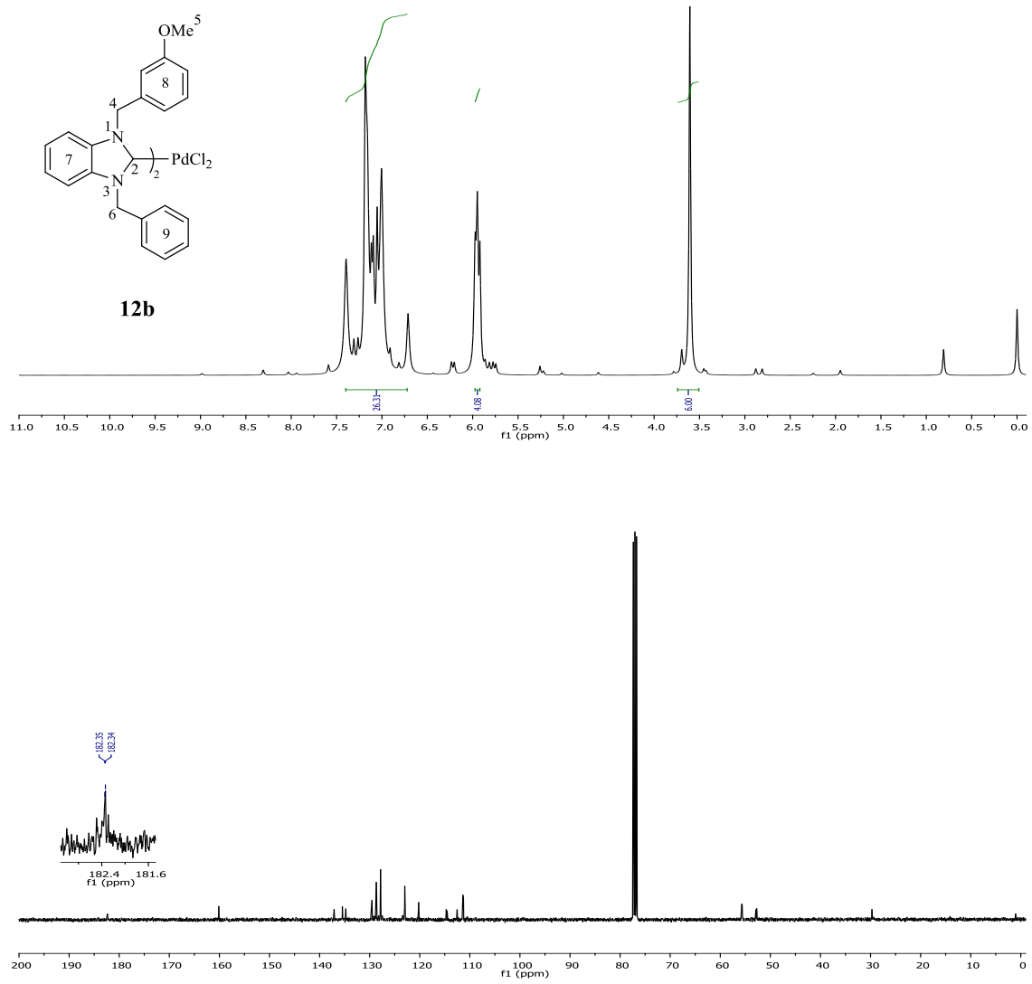
Şekil 3.65 12b Bileşiğine ait 1 H ve 13 C NMR spektrumları.
