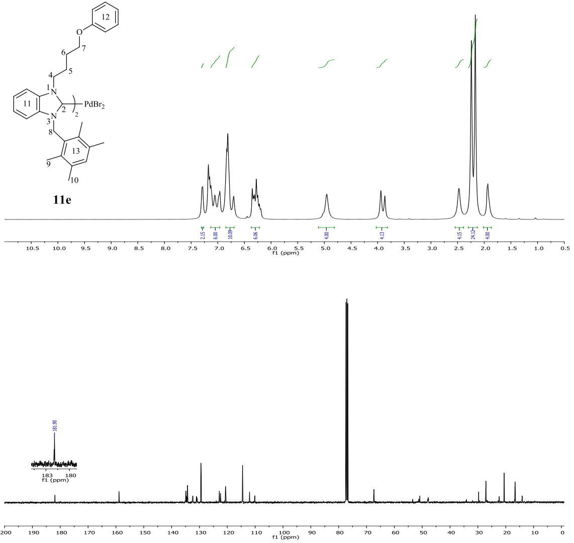
Şekil 3.61 11e Bileşiğine ait 1 H ve 13 C NMR spektrumları.
