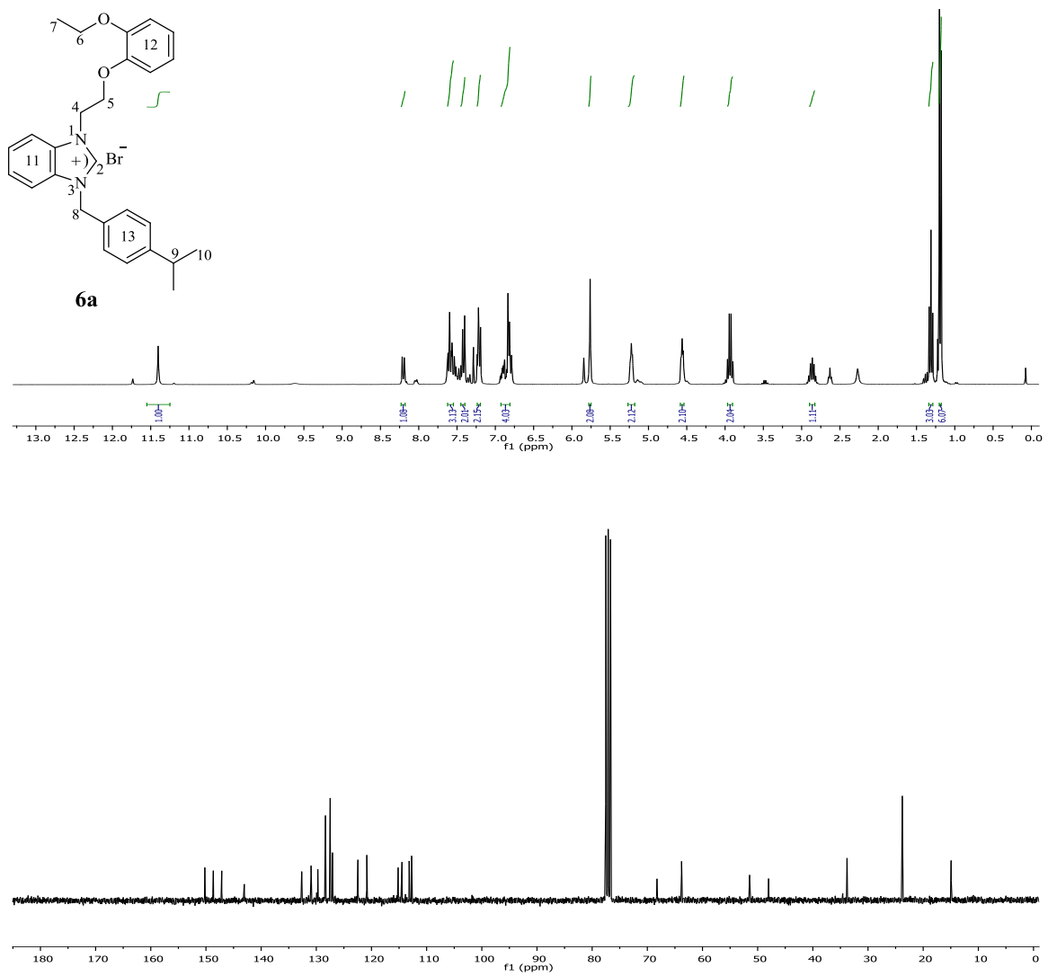
Şekil 3.32 6a Bileşiğine ait 1 H ve 13 C NMR spektrumları.
