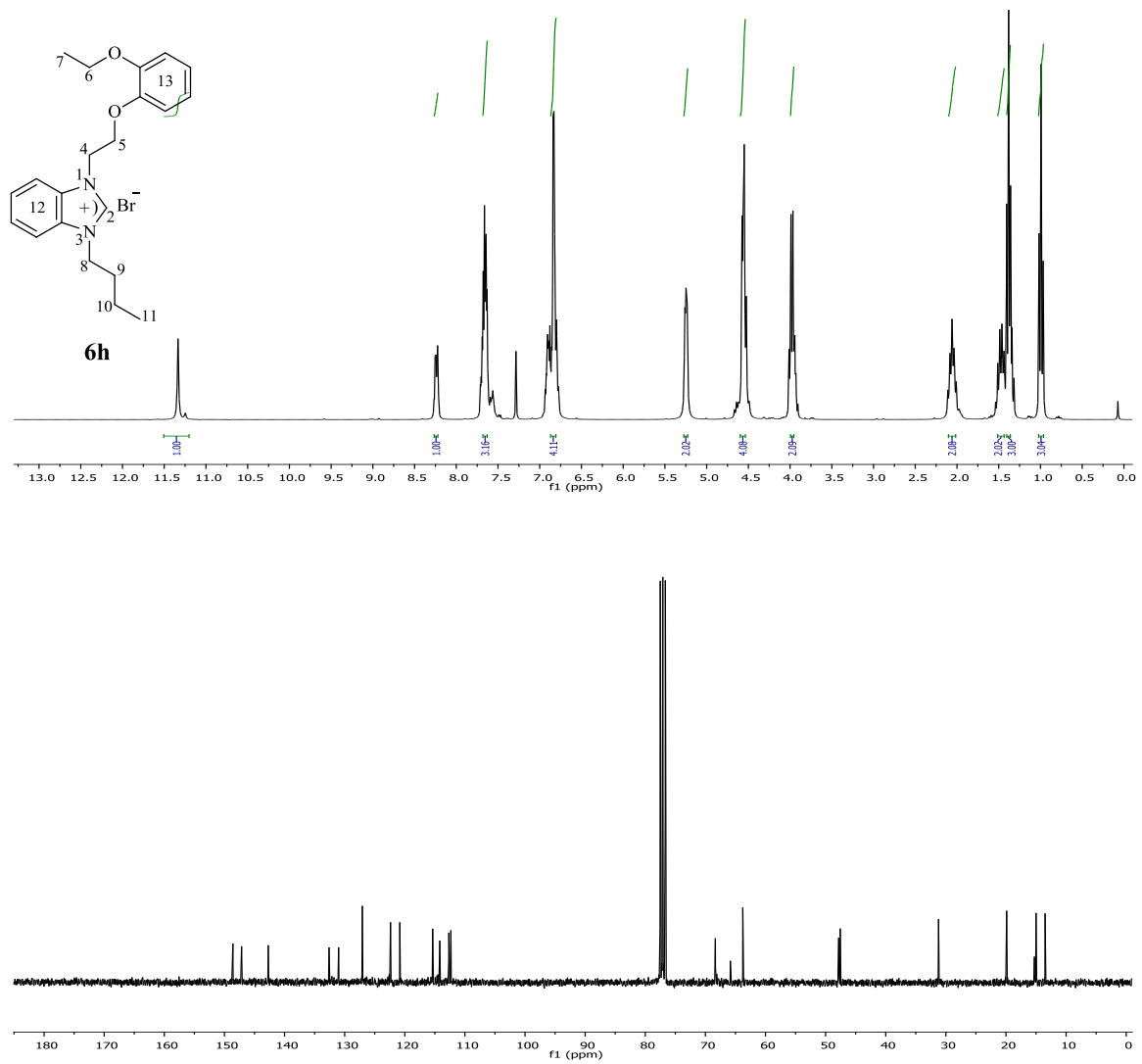
Şekil 3.35 6h Bileşiğine ait 1 H ve 13 C NMR spektrumları.
