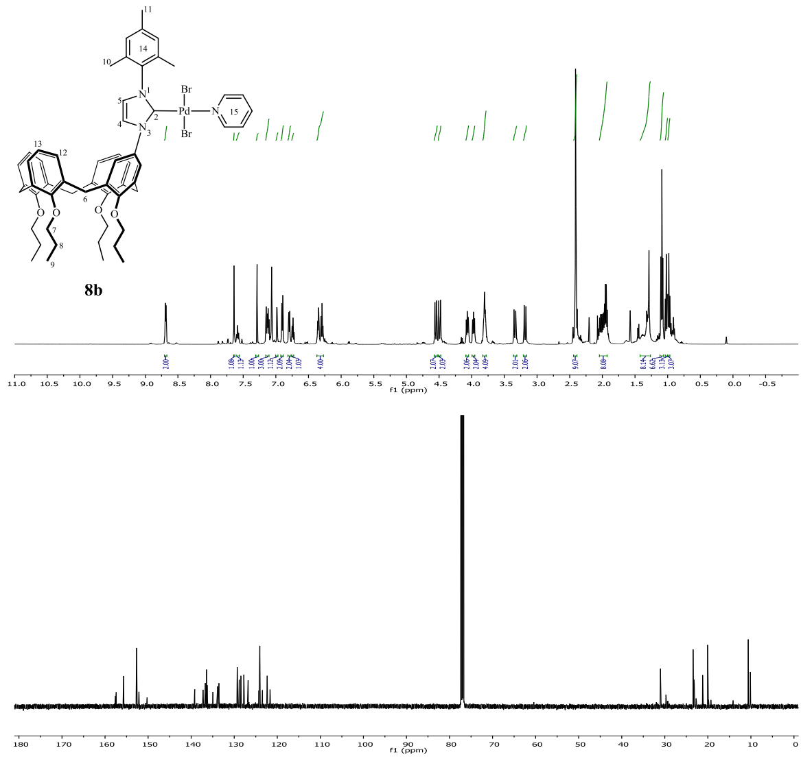
Şekil 3.40 8b Bileşiğine ait 1 H ve 13 C NMR spektrumları.
