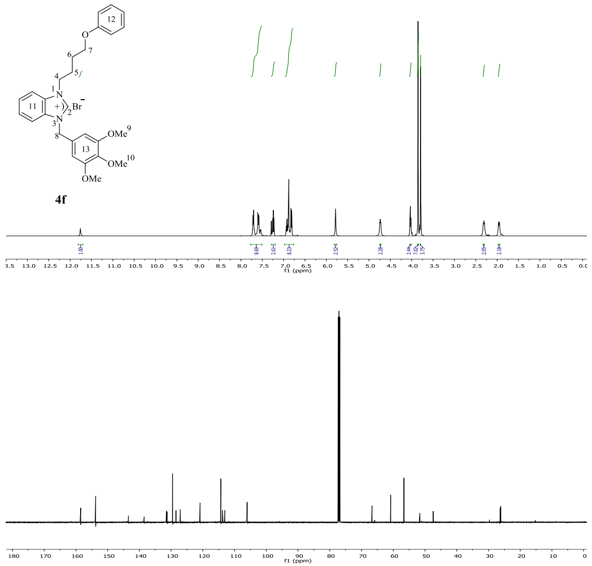
Şekil 3.23 4f Bileşiğine ait ^1\text{H} ve ^{13}\text{C} NMR spektrumları.
