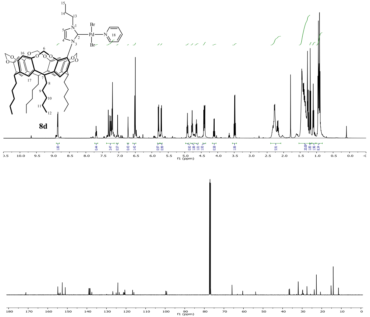
Şekil 3.42 8d Bileşiğine ait ^1\text{H} ve ^{13}\text{C} NMR spektrumları.
