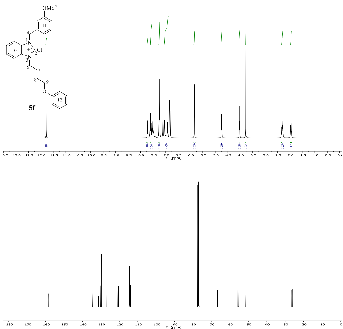
Şekil 3.31 5f Bileşiğine ait 1 H ve 13 C NMR spektrumları.
