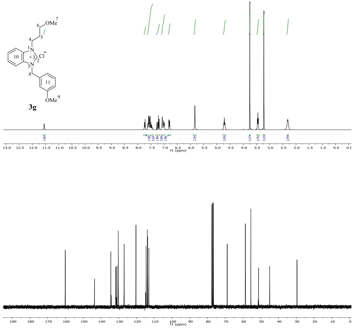
Şekil 3.14 3g Bileşiğine ait 1 H ve 13 C NMR spektrumları.
