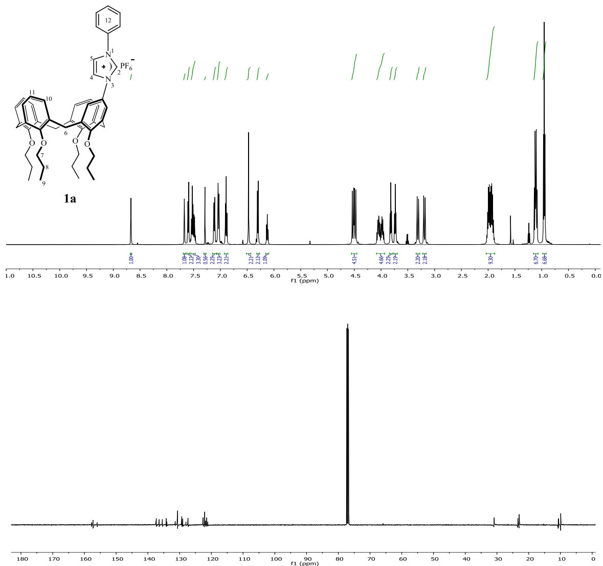
Şekil 3.1 1a Bileşiğine ait ^1\text{H} ve ^{13}\text{C} NMR spektrumları.
