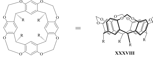
Şekil 1.18 Metilendioksi köprülü resorsin[4]aren kavitanı.
