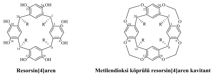
Şekil 1.20 Resorsin[4]aren halkasının numaralandırılması.
