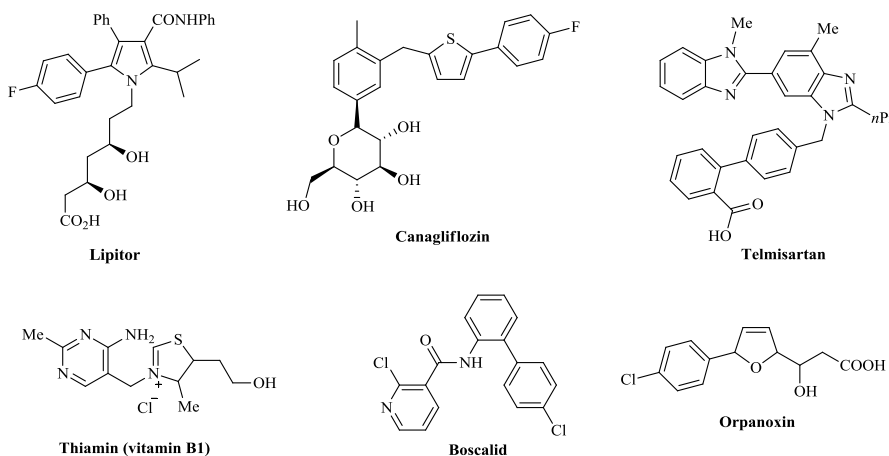
Şekil 1.12 Endüstriyel açıdan önemli bazı bi(hetero)aril bileşikler.
