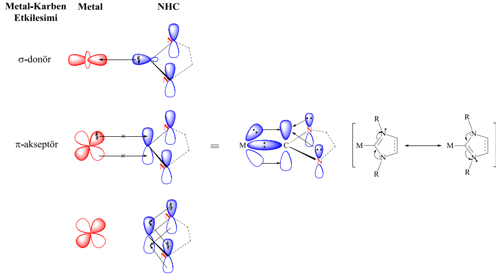
Şekil 1.10 N-Heterosiklik karben komplekslerinde bağlanma ve rezonans yapıları.
