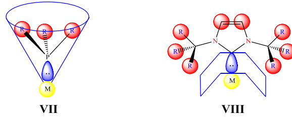
Şekil 1.6 Fosfin ve NHC ligandlarının metal merkezi üzerindeki sterik etkisi.
