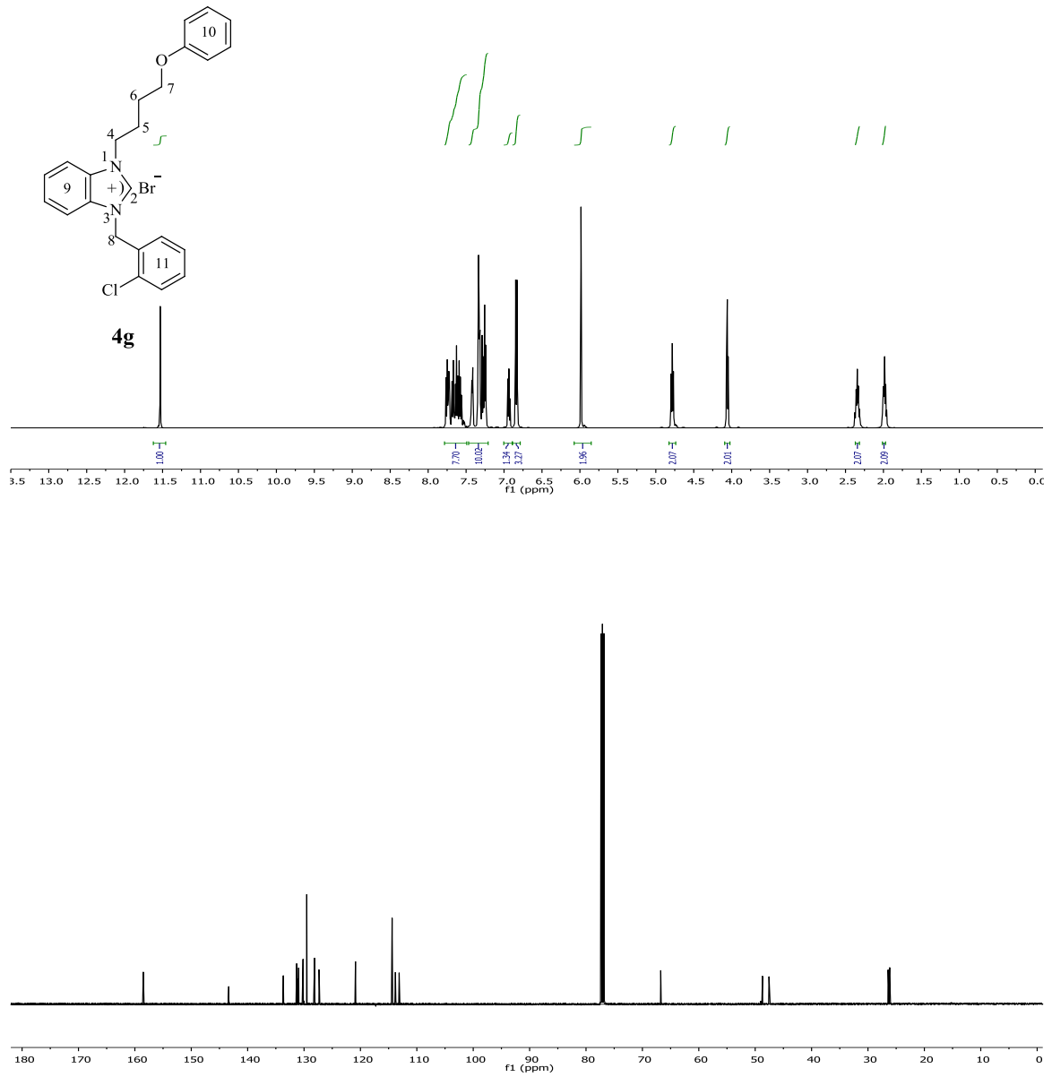
Şekil 3.24 4g Bileşiğine ait 1 H ve 13 C NMR spektrumları.
