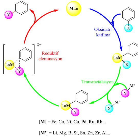
Şema 1.3 Geçiş-metal katalizli çapraz eşleşme tepkimelerine ait katalitik çevrim.
