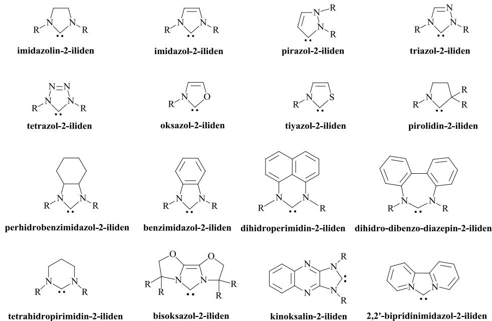
Şekil 1.4 Günümüze kadar sentezlenen bazı önemli N -heterosiklik karben türleri.
