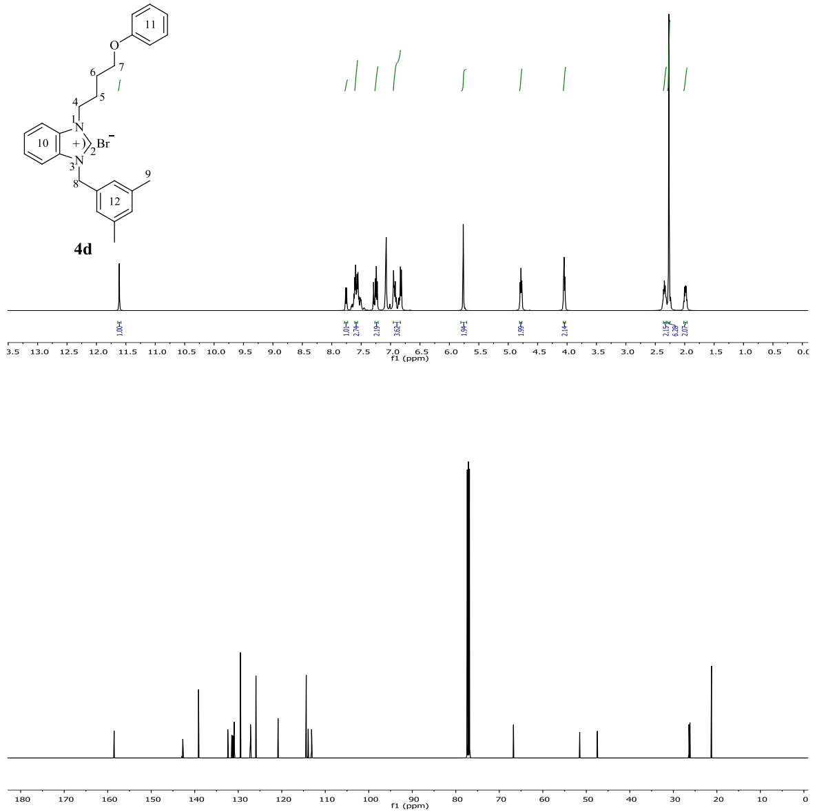
Şekil 3.21 4d Bileşiğine ait ^1\text{H} ve ^{13}\text{C} NMR spektrumları.
