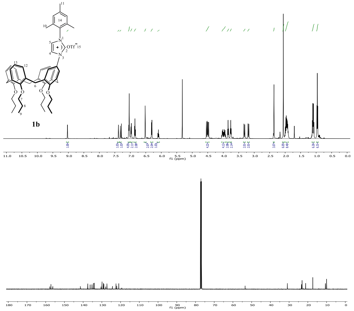
Şekil 3.3 1b Bileşiğine ait 1 H ve 13 C NMR spektrumları.
