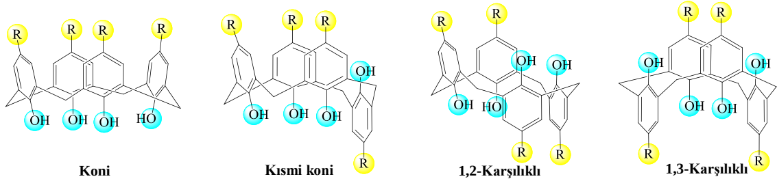
Şekil 1.15 Tetramerik yapıdaki kaliks[4]aren halkasına ait konformasyonlar.
