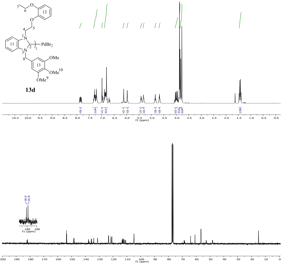
Şekil 3.73 13d Bileşiğine ait 1 H ve 13 C NMR spektrumları.
