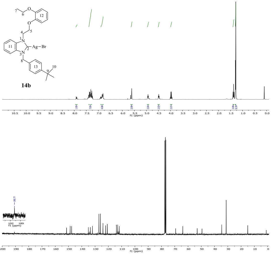
Şekil 3.77 14b Bileşiğine ait 1 H ve 13 C NMR spektrumları.
