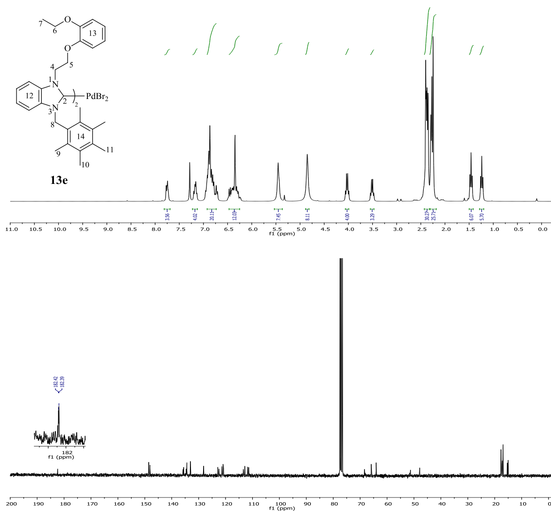
Şekil 3.74 13e Bileşiğine ait 1 H ve 13 C NMR spektrumları.
