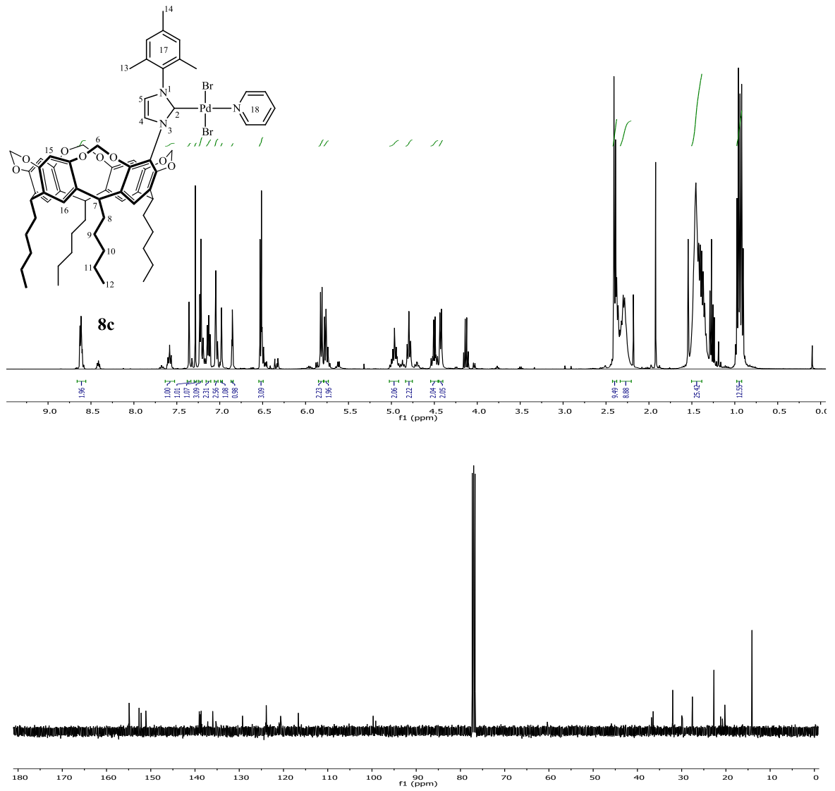
Şekil 3.41 8c Bileşiğine ait ^1\text{H} ve ^{13}\text{C} NMR spektrumları.
