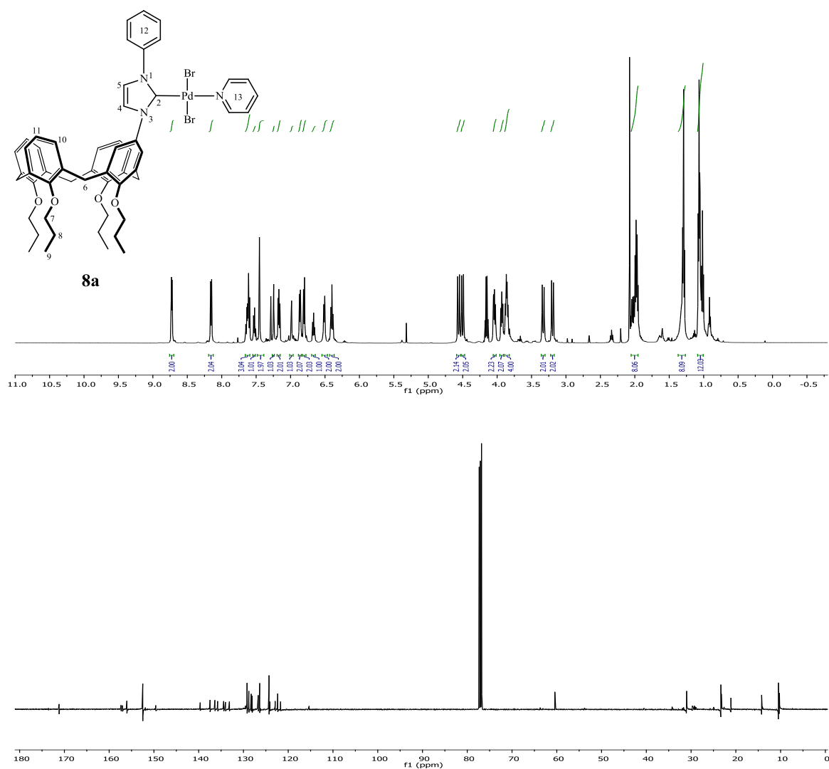
Şekil 3.39 8a Bileşiğine ait 1 H ve 13 C NMR spektrumları.
