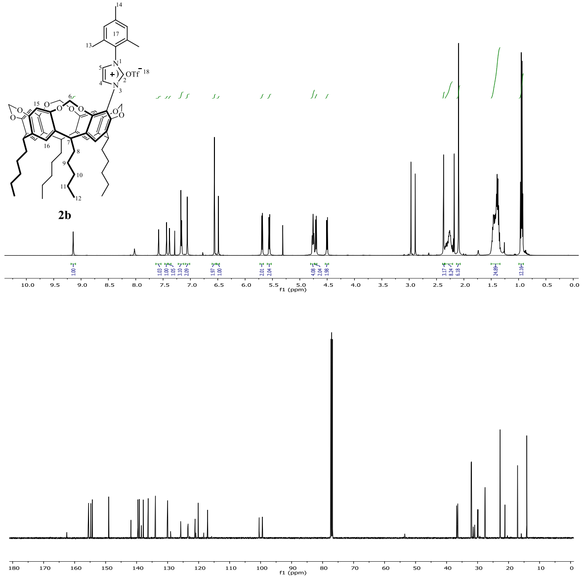
Şekil 3.6 2b Bileşiğine ait ^1\text{H} ve ^{13}\text{C} NMR spektrumları.
