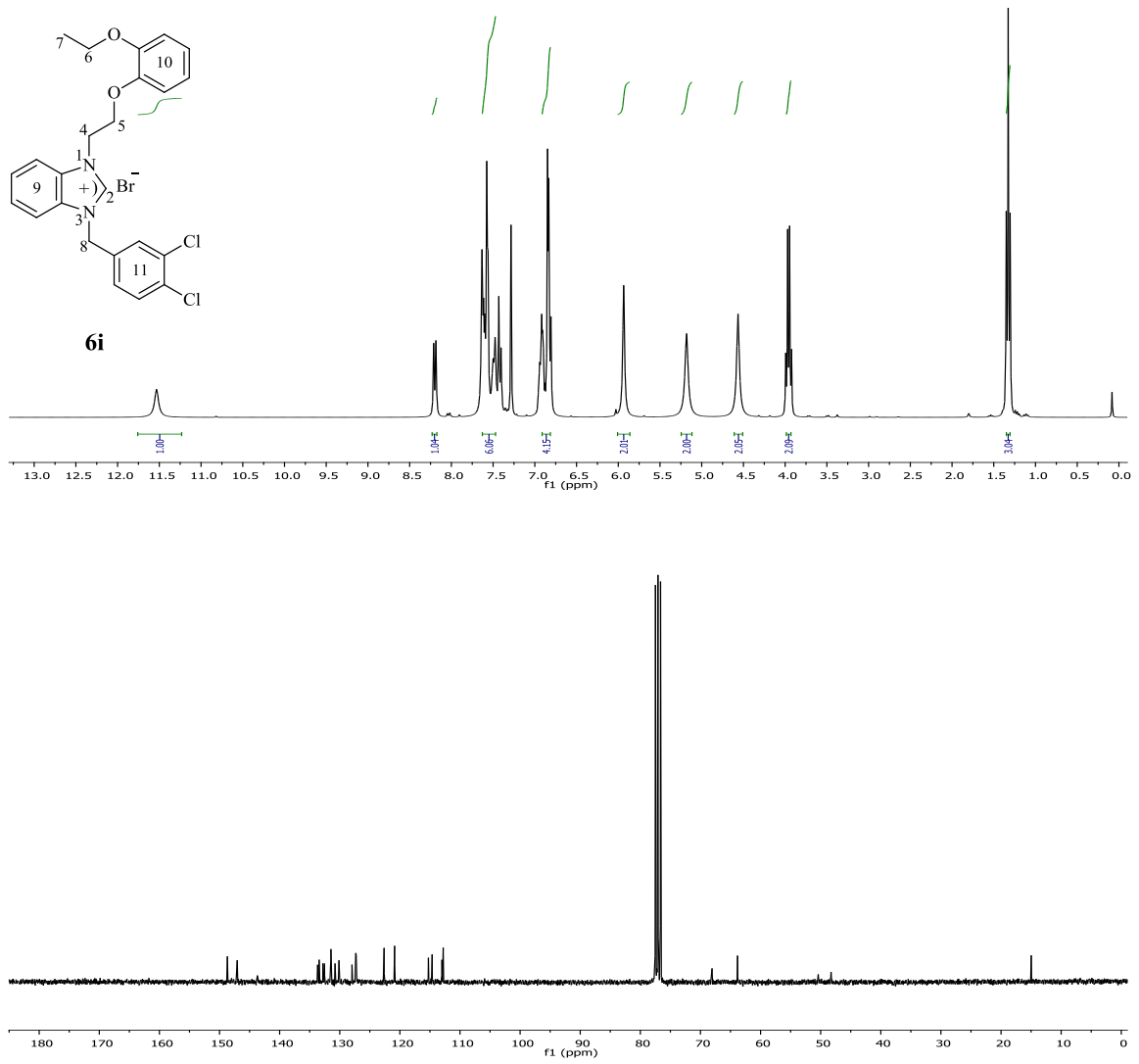
Şekil 3.36 6i Bileşiğine ait ^1\text{H} ve ^{13}\text{C} NMR spektrumları.
