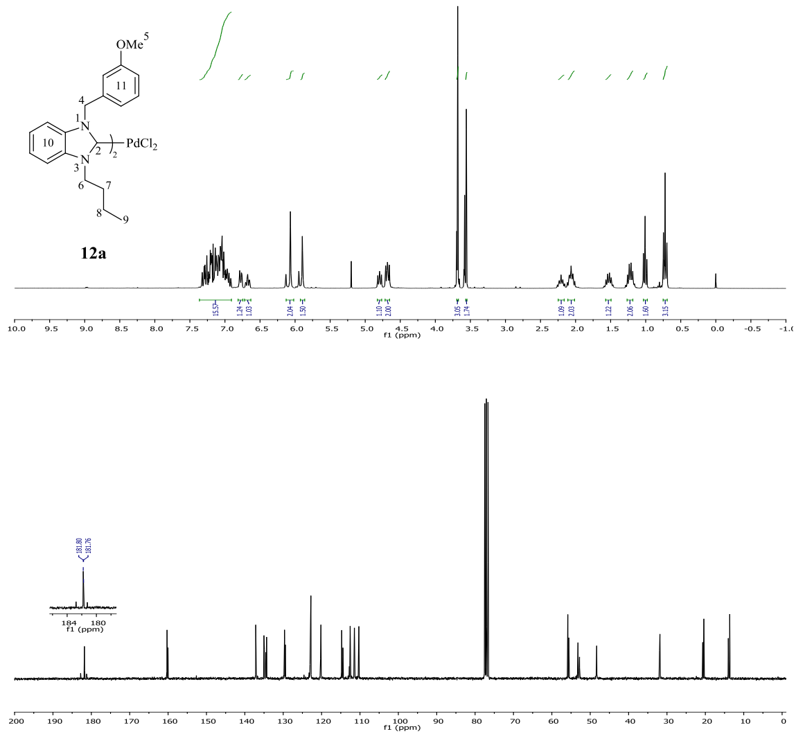
Şekil 3.64 12a Bileşiğine ait 1 H ve 13 C NMR spektrumları.
