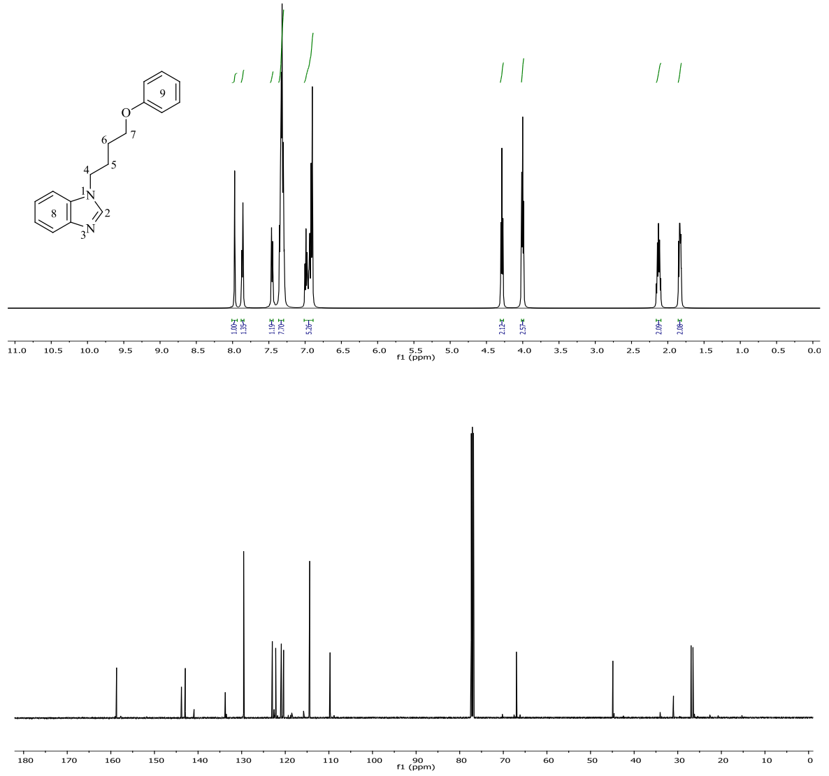
Şekil 3.17 N -(4-Fenoksibütıl)benzimidazol bileşiğine ait ^1\text{H} ve ^{13}\text{C} NMR spektrumları.
