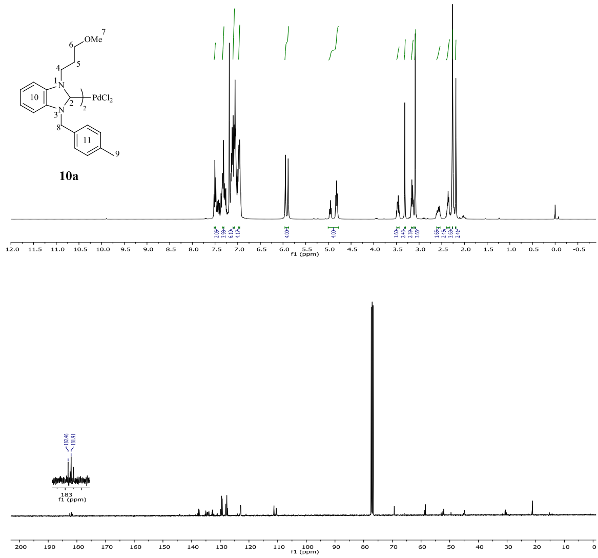
Şekil 3.50 10a Bileşiğine ait 1 H ve 13 C NMR spektrumları.
