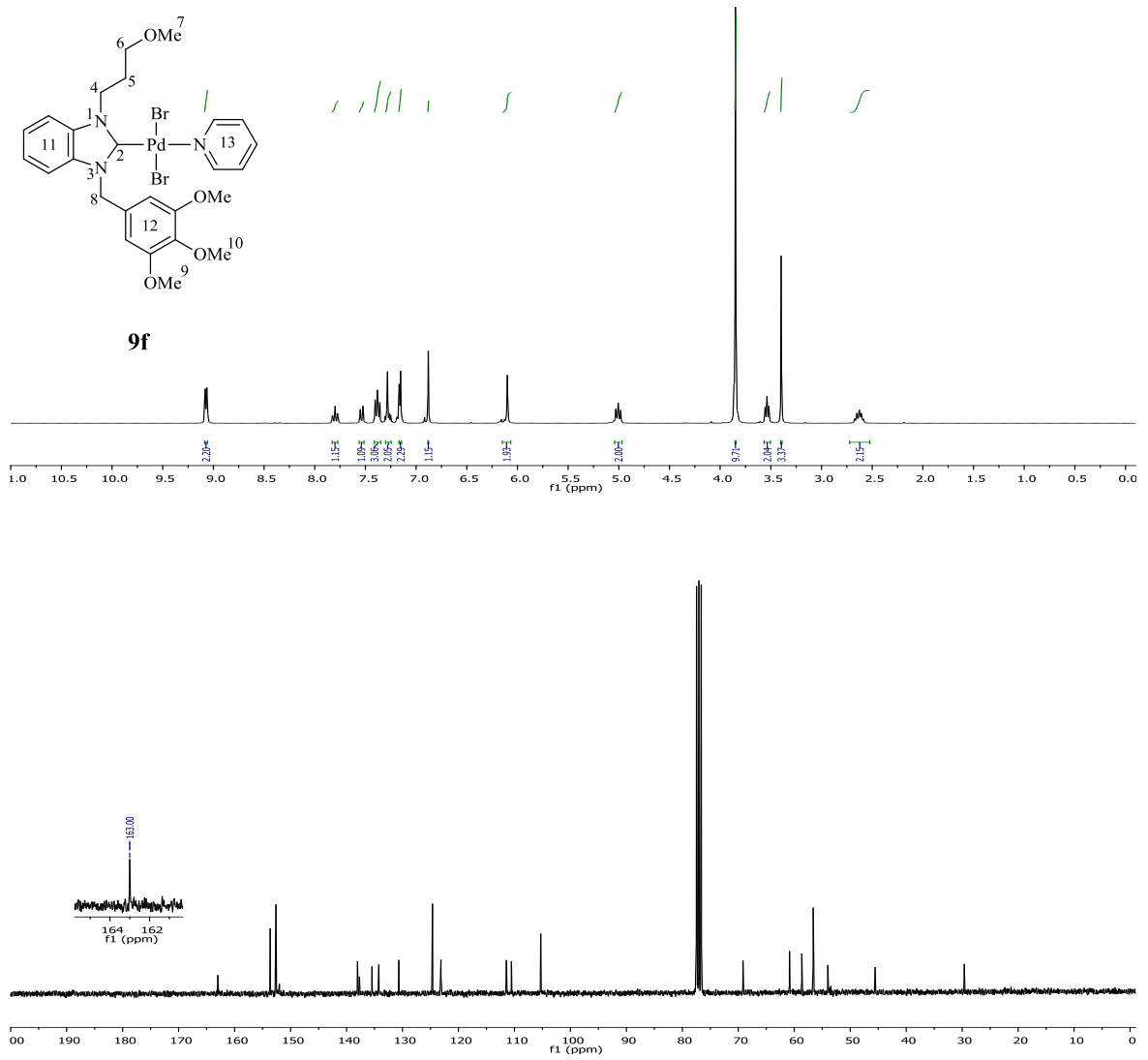
Şekil 3.48 9f Bileşiğine ait 1 H ve 13 C NMR spektrumları.
