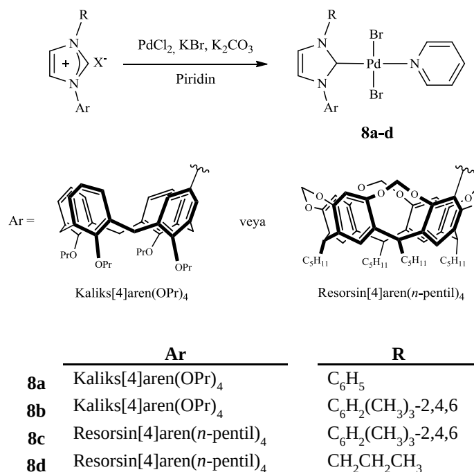
Şema 3.7 Sentezlenen kaliks[4]aren ve resorsin[4]aren sübstitüye Pd-NHC-PEPPSI kompleksleri.
