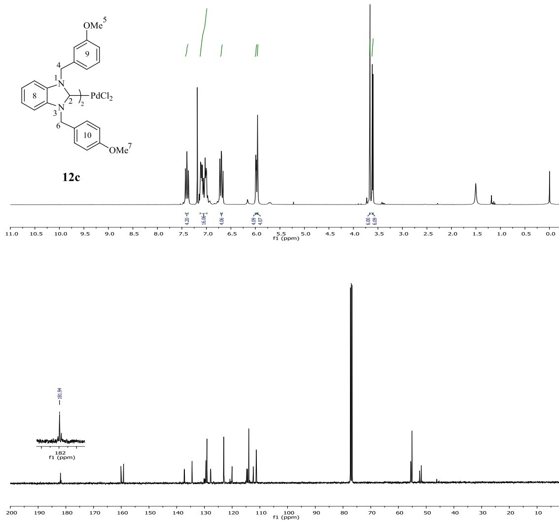
Şekil 3.66 12c Bileşiğine ait 1 H ve 13 C NMR spektrumları.
