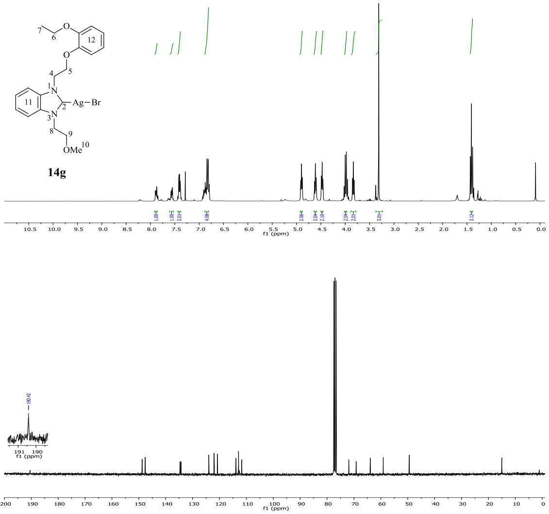
Şekil 3.82 14g Bileşiğine ait 1 H ve 13 C NMR spektrumları.
