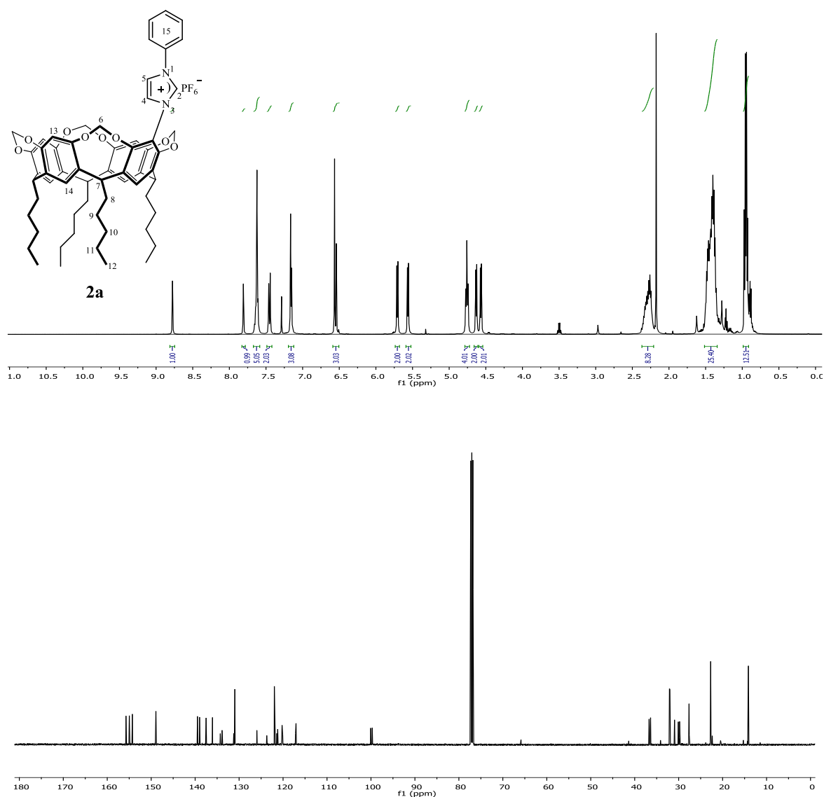
Şekil 3.5 2a Bileşiğine ait 1 H ve 13 C NMR spektrumları.
