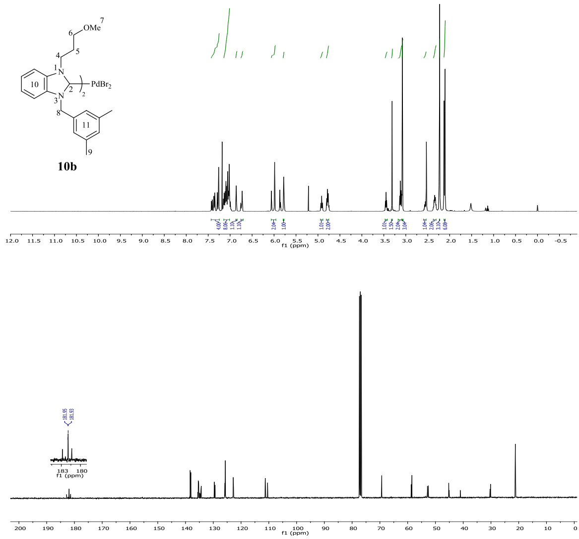
Şekil 3.51 10b Bileşiğine ait 1 H ve 13 C NMR spektrumları.
