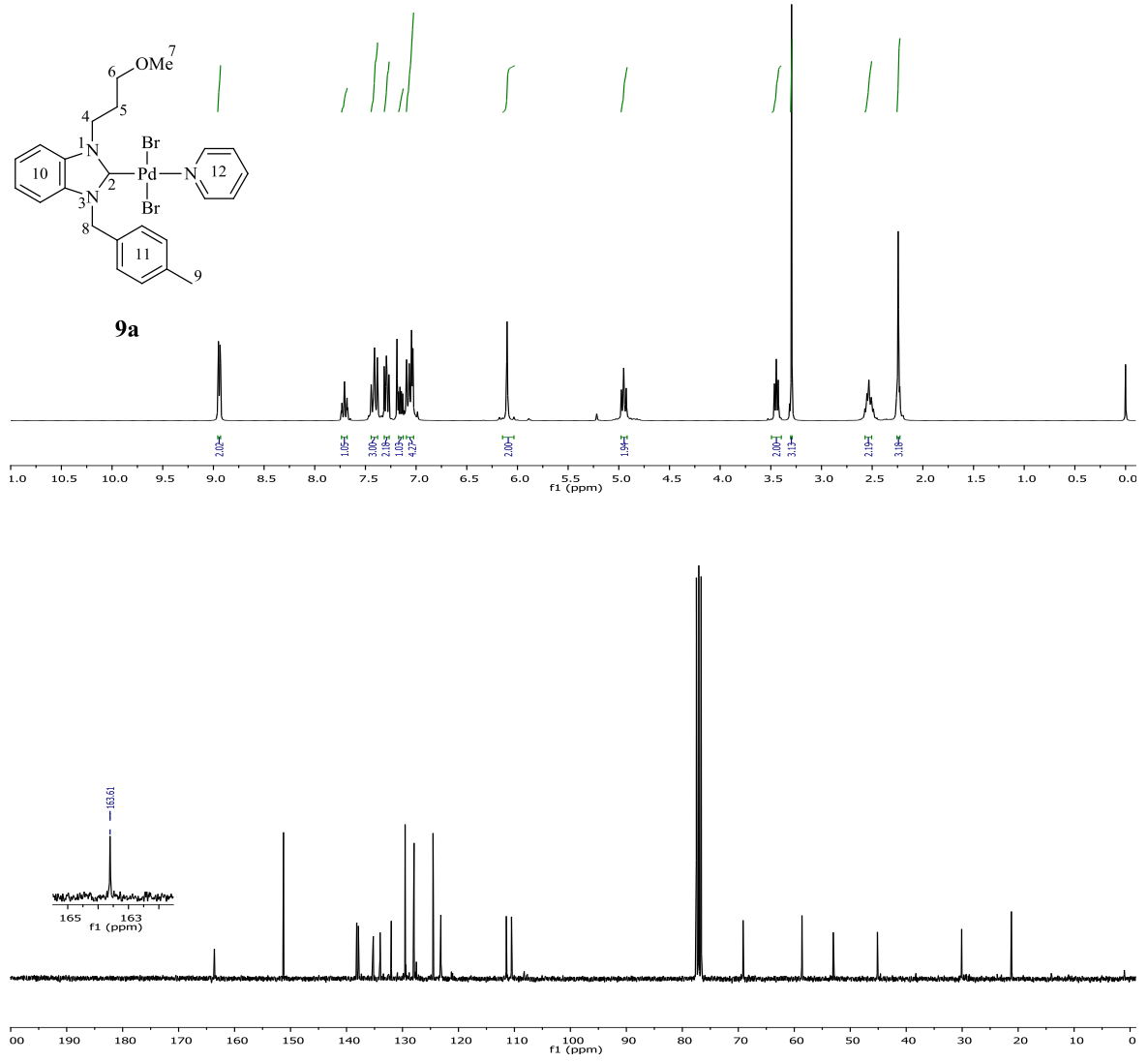
Şekil 3.43 9a Bileşiğine ait 1 H ve 13 C NMR spektrumları.
