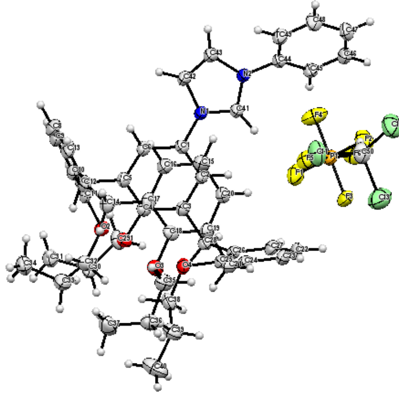
Şekil 3.2 1a Bileşiğinin X-ışını yapısı.
