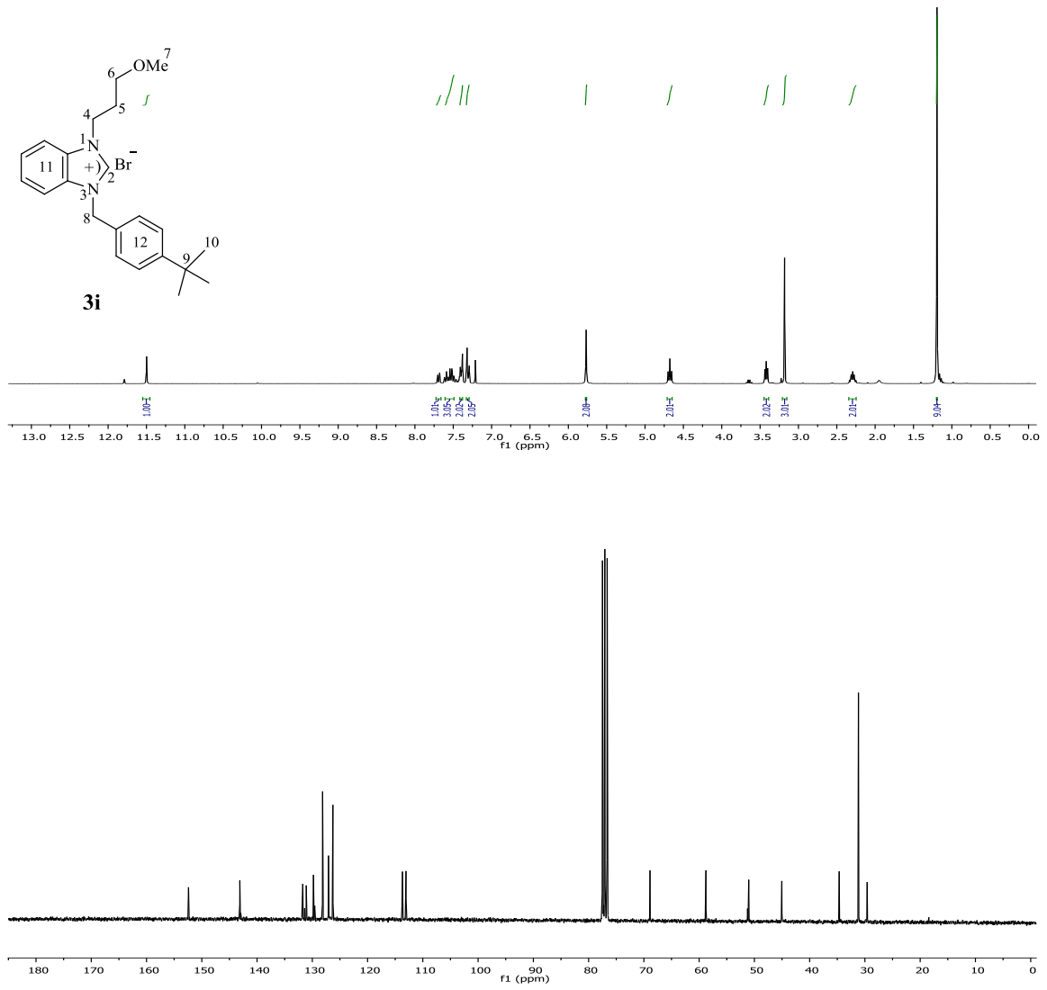
Şekil 3.16 3i Bileşiğine ait 1 H ve 13 C NMR spektrumları.
