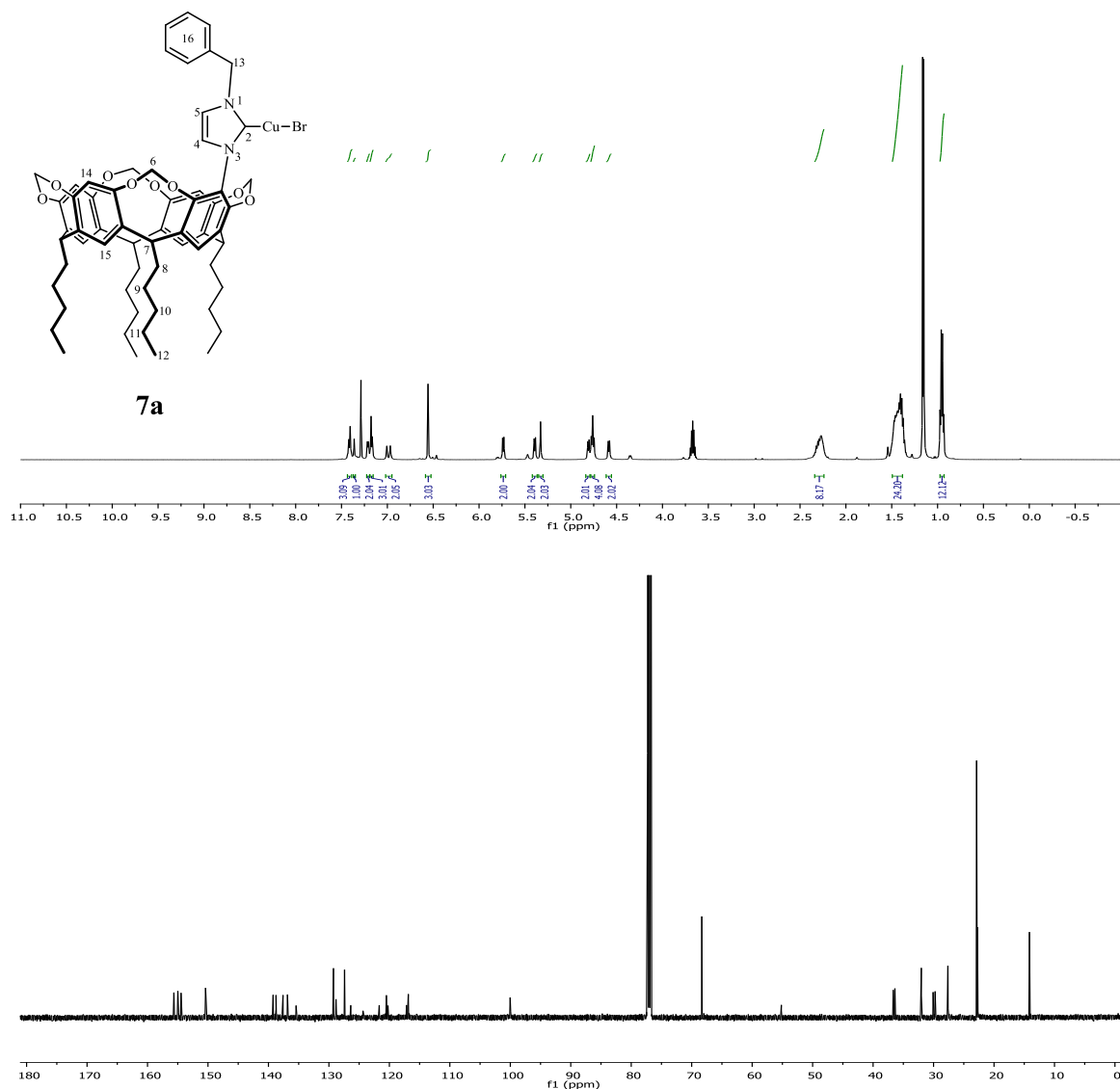
Şekil 3.37 7a Bileşiğine ait 1 H ve 13 C NMR spektrumları.
