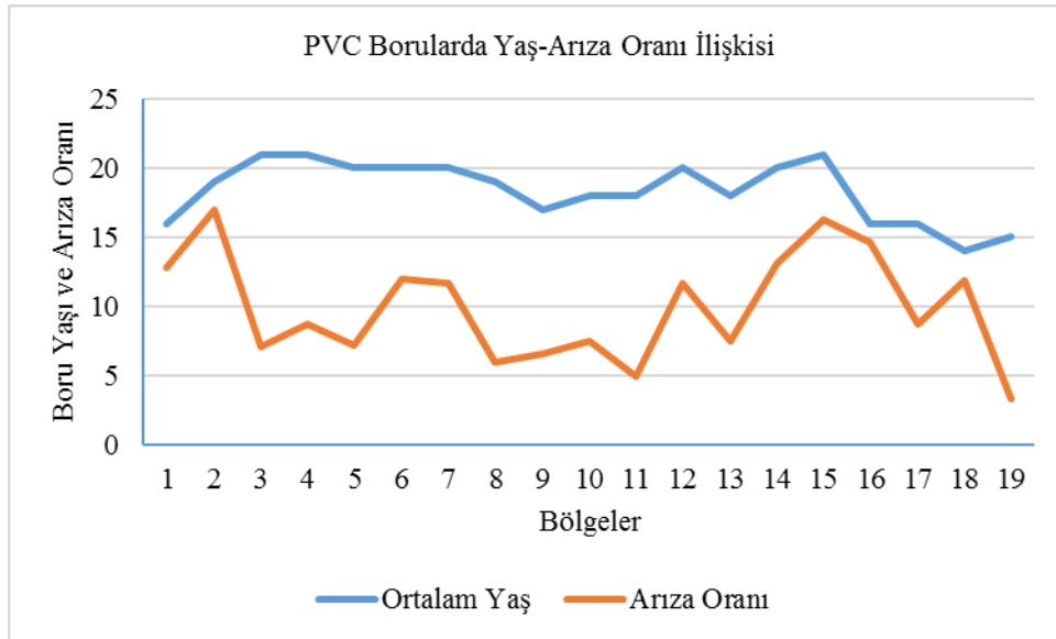
Şekil 5.32. PVC borularda yaş ve arıza oranı ilişkisi
