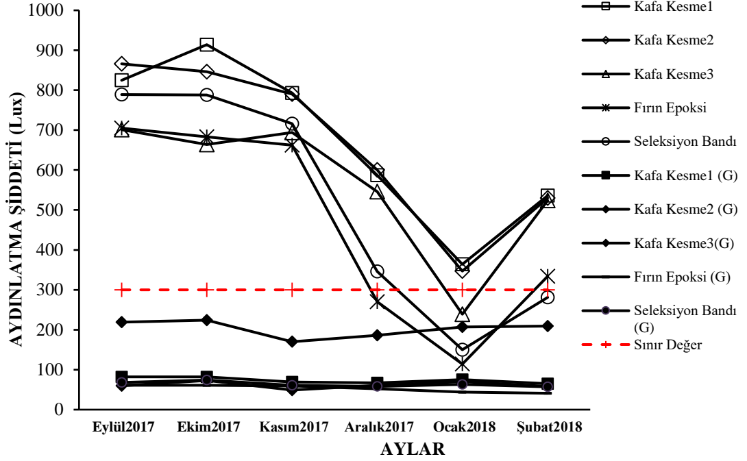
Şekil 4.1. Mermer kesim tesisinde aylara göre değişen aydınlatma ölçüm sonuçları
