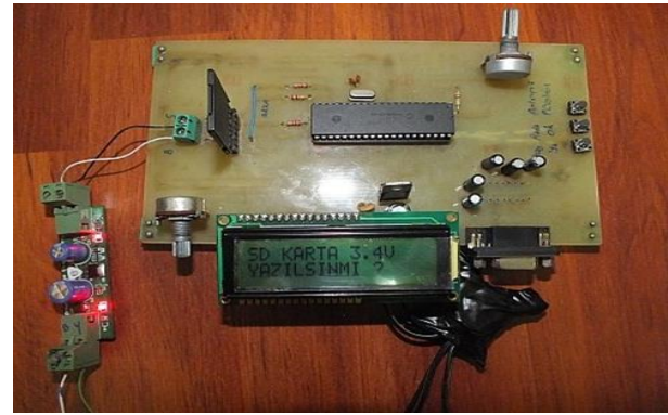
Şekil 5: Çalışma için geliştirilen elektronik kart
